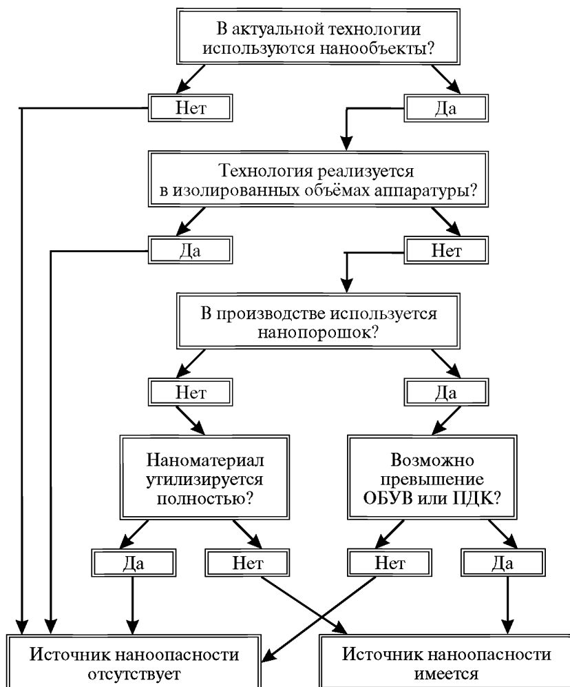
Рис. 2. Алгоритм установления источника опасности на предприятии nanoиндустрии
