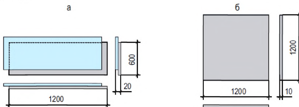
а – элемент пола; б – влагостойкий гипсоволокнистый лист ГВЛВ
