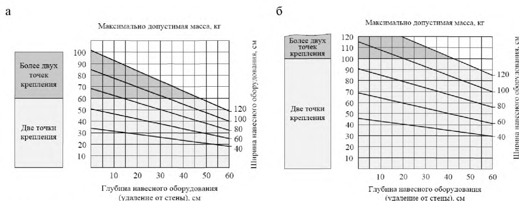
Рисунок 11 – Графики для определения допустимой массы навесного оборудования высотой более 30 см при консольной нагрузке на перегородку
