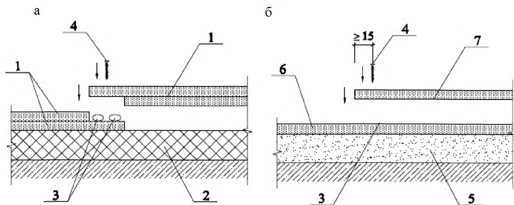
а – соединение ЭП; б – соединение малоформатных ГВЛВ 1 – элемент пола; 2 – тепло- звукоизоляционный материал; 3 – клеящая мастика; 4 – винт для ГВЛВ; 5 – сухая засыпка; 6 – ГВЛВ первого слоя; 7 – ГВЛВ второго слоя
