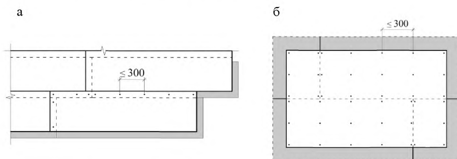
а – крепление ЭП; б – крепление малоформатных ГВЛВ
