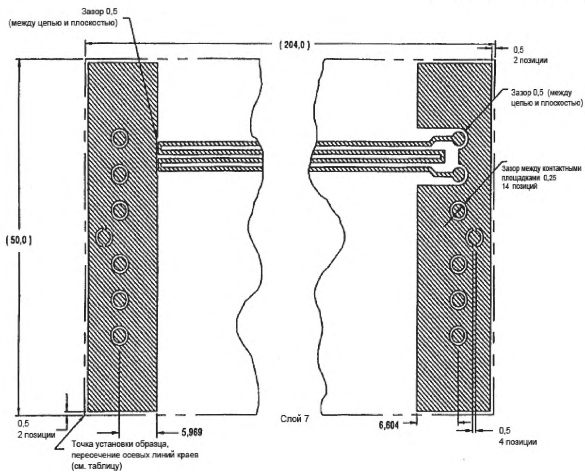
Рисунок 1I – Образцы для испытания H2 и H3 – продолжение
