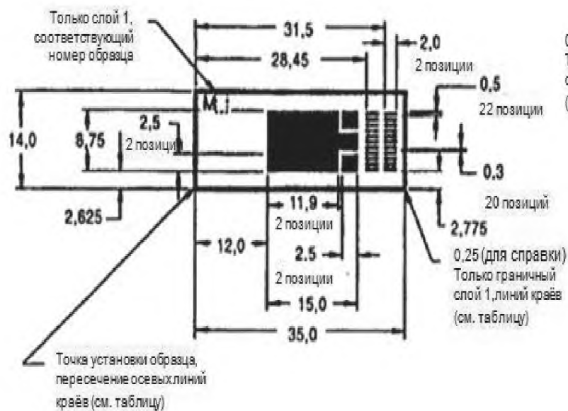
Рисунок 1m— Образцы для испытания L и M
