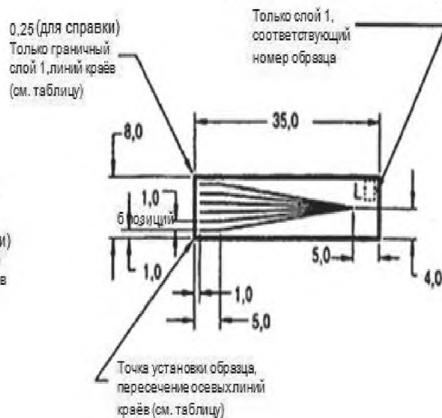
Рисунок 1m— Образцы для испытания L и M
