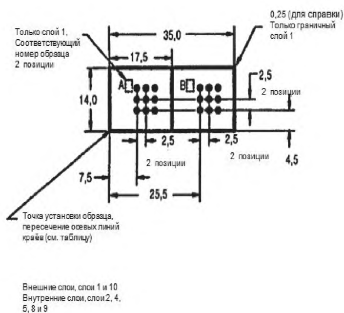
Рисунок 1а – Образцы для испытания А и В
