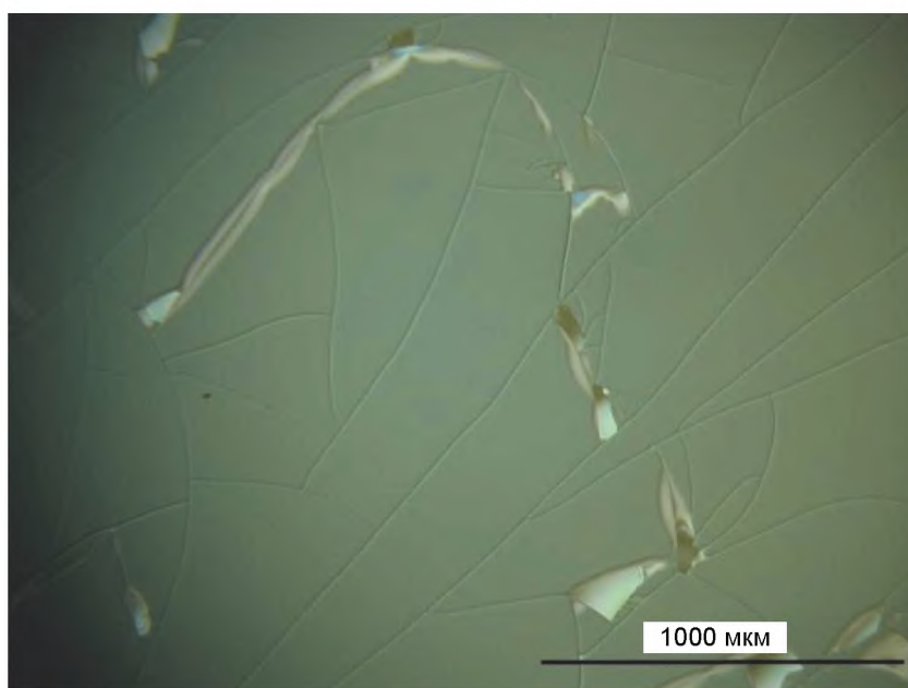
Рисунок А.8 – Трещина
