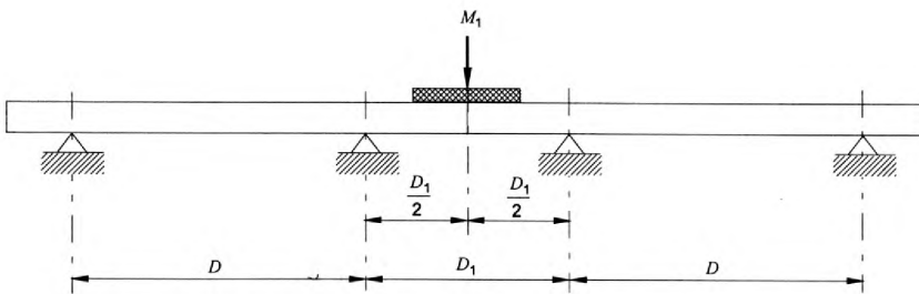
Рисунок 5 – Испытание прямых секций статической нагрузкой
