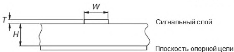
Рисунок 4 – Поверхностная микрополосковая линия
