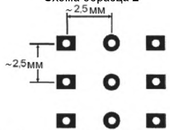
Единичный тест-купон волнового сопротивления Схема образца 2
