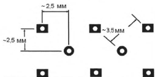
Единичный тест-купон волнового сопротивления Схема образца 1А
