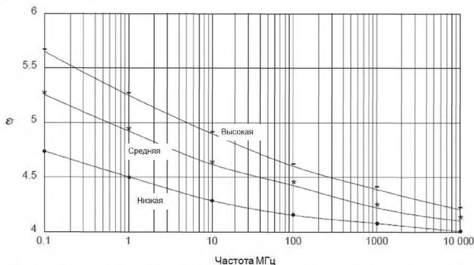
Рисунок 2 – Зависимость \varepsilon_r от частоты (слоистый материал эпоксидная смола/стекло)
