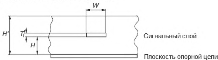
Рисунок 5 – Встроенная микрополосковая линия
