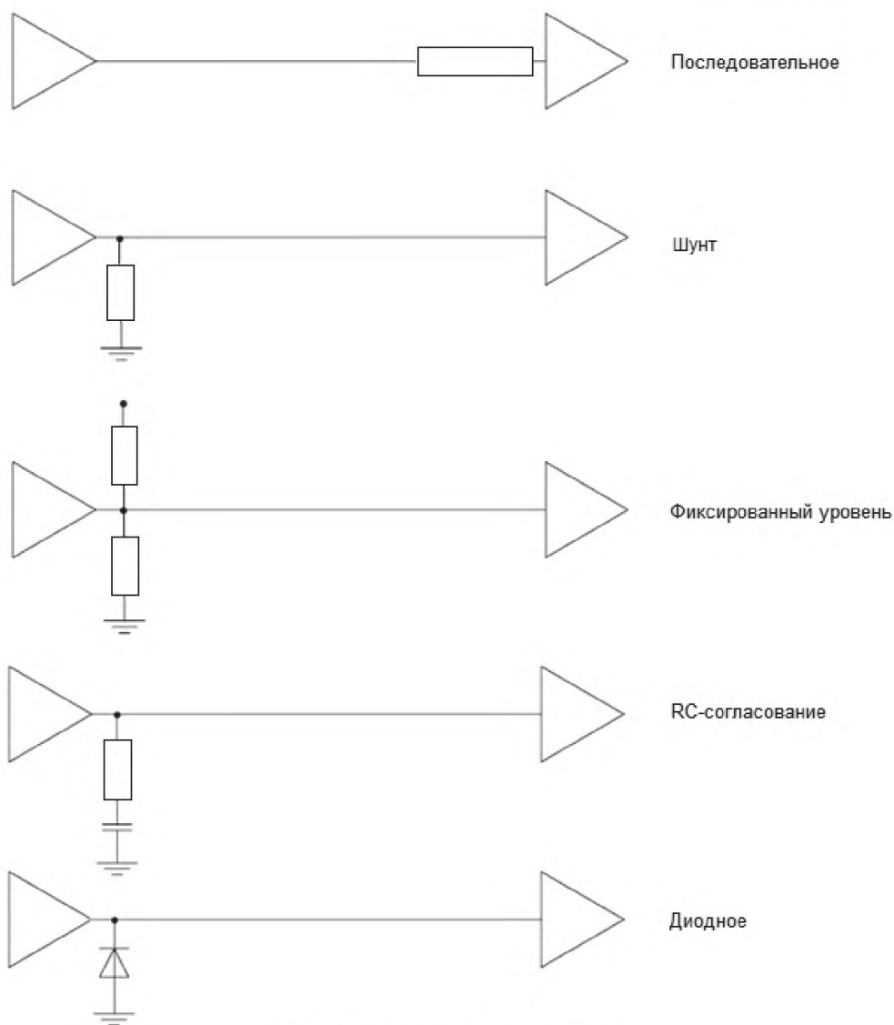
Рисунок 3 – Согласование нагрузок
