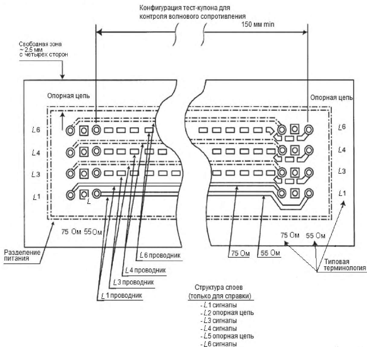
Рисунок 10 – Тест-купон контролируемого волнового сопротивления
