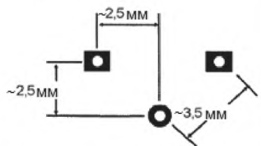
Единичный тест-купон волнового сопротивления Схема образца 1В
