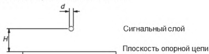
Рисунок 9 – Микрополосковая проводная линия
