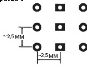
Единичный тест-купон волнового сопротивления Схема образца 3
