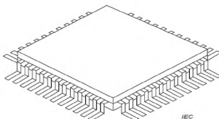
Рисунок 9 — корпус типа PLQFP (квадратный)
