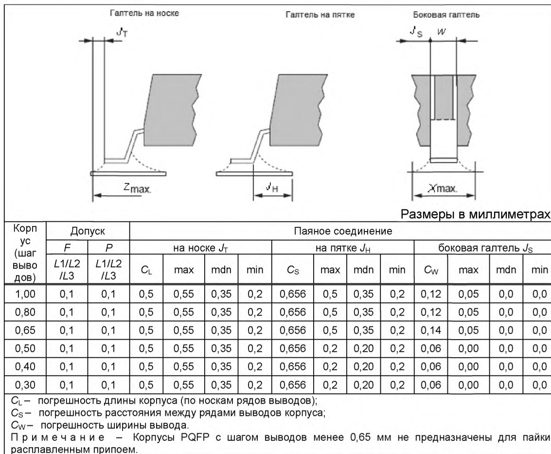
Рисунок 3 — Анализ формы паяного соединения
