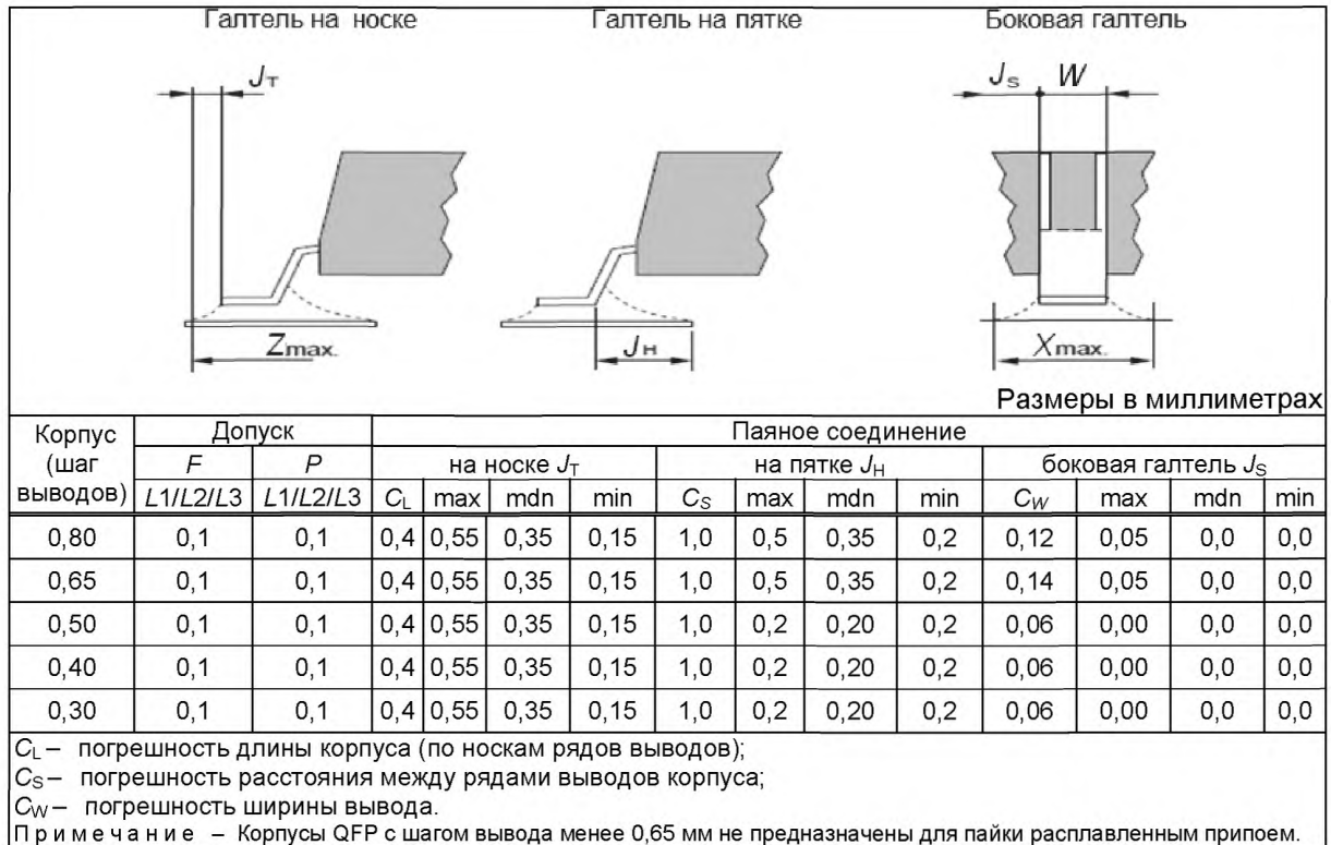
Рисунок 11 – Анализ формы паяного соединения
