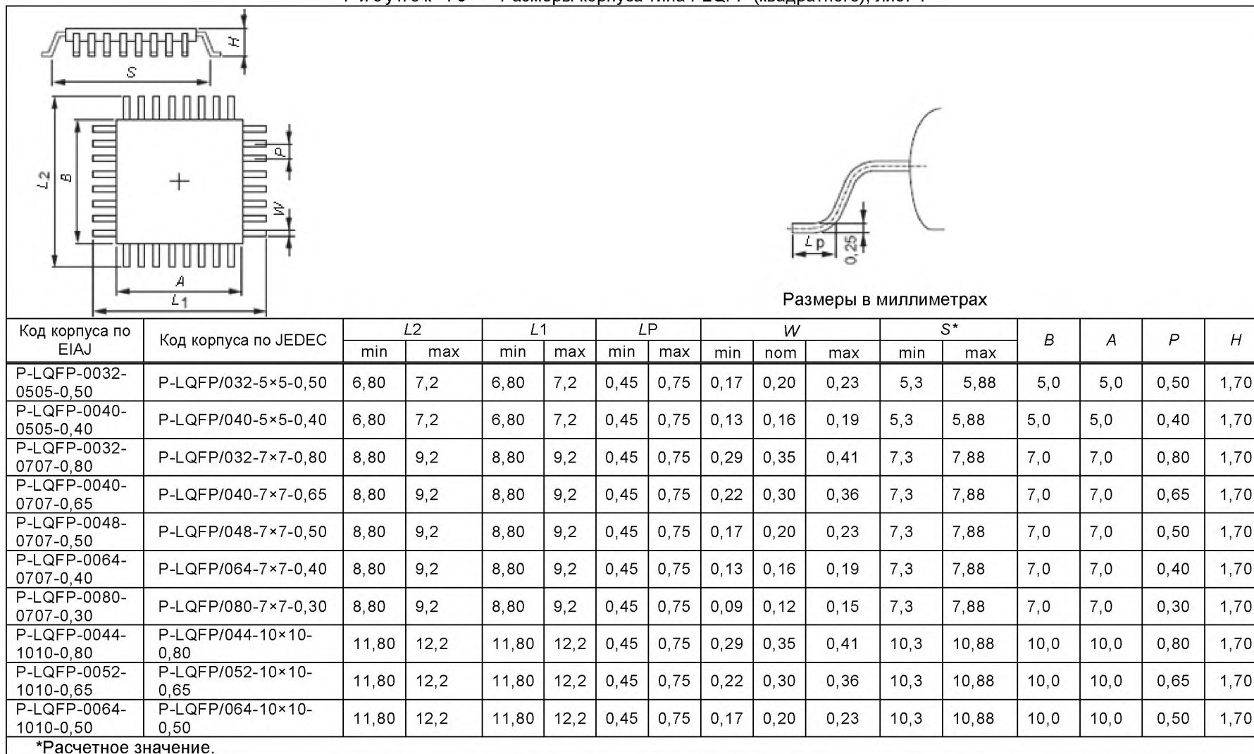
Рисунок 10 – Размеры корпуса типа PLQFP (квадратного), лист 1
