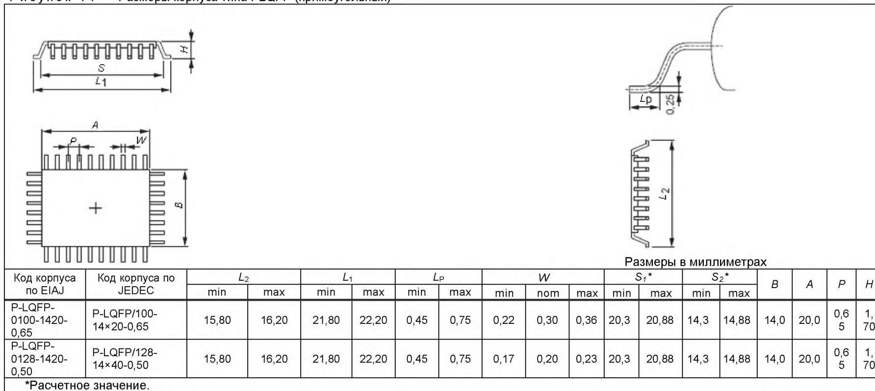
Рисунок 14 – Размеры корпуса типа PLQFP (прямоугольный)
