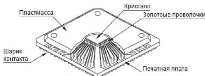
Рисунок 4 – Корпус BGA (квадратный)
