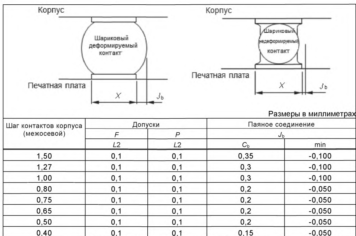
Рисунок 6 – Анализ формы паяного соединения
