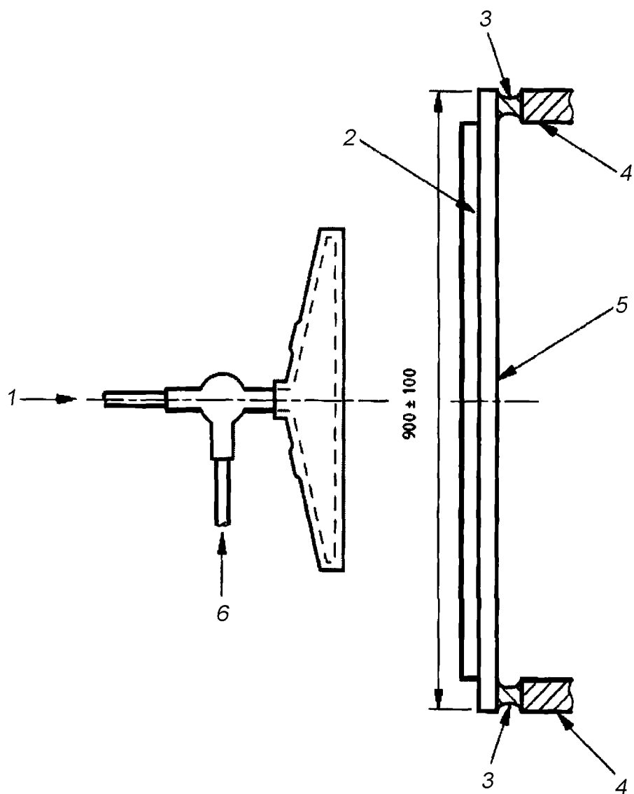
1 — подача воздуха; 2 — панель; 3 — резиновая втулка; 4 — стальная опора; 5 — горизонтальная стальная опора для панели; 6 — подача пропана
