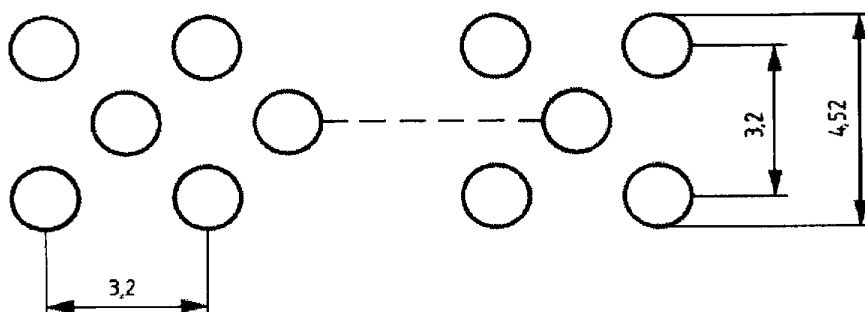
Рисунок 5 — Фронтальная поверхность рабочей части горелки
