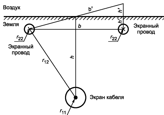
Рисунок В.2 — Принцип применения двух экранирующих проводов
