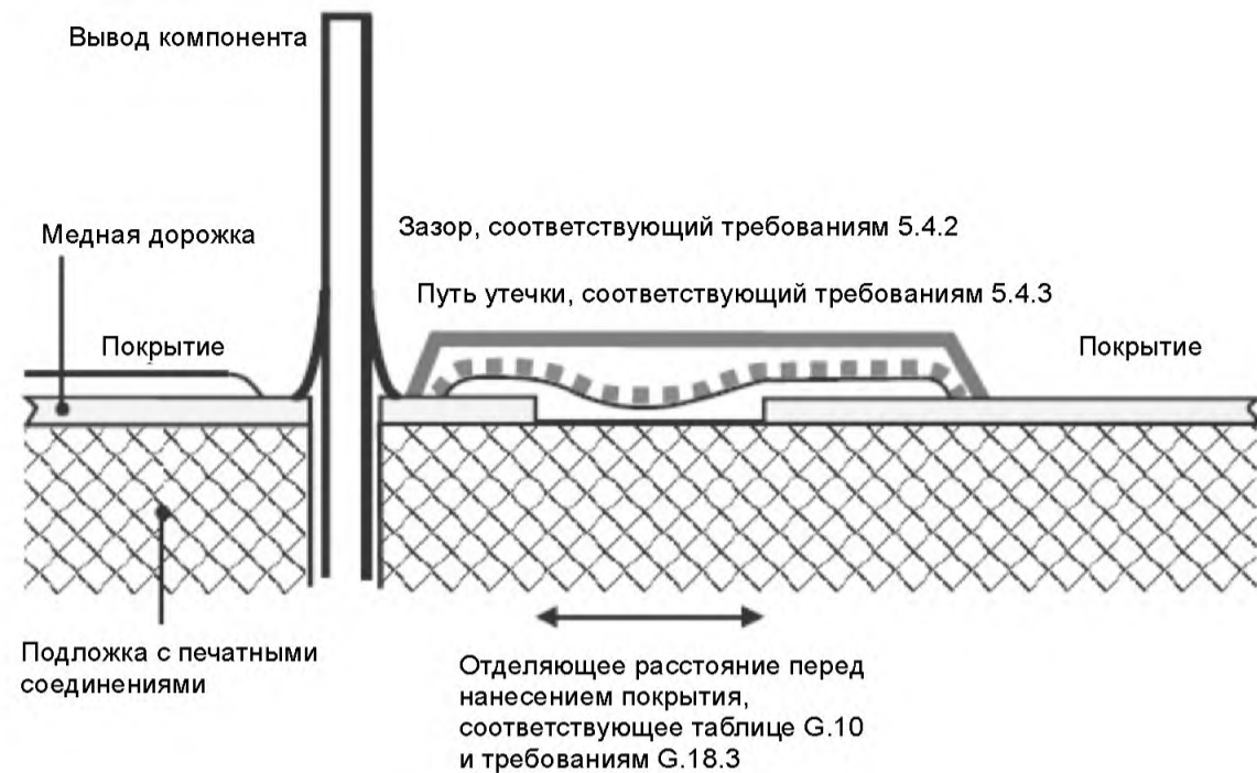
Рисунок О.12 — Покрытие поверх печатного монтажа
