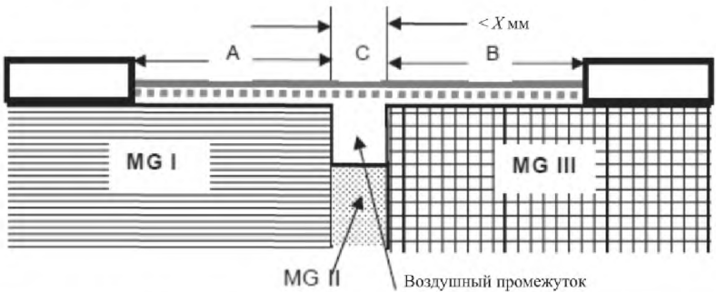
Рисунок О.18 — Компоненты из материалов с разными значениями СИТ, воздушный промежуток между которыми имеет ширину менее X мм
