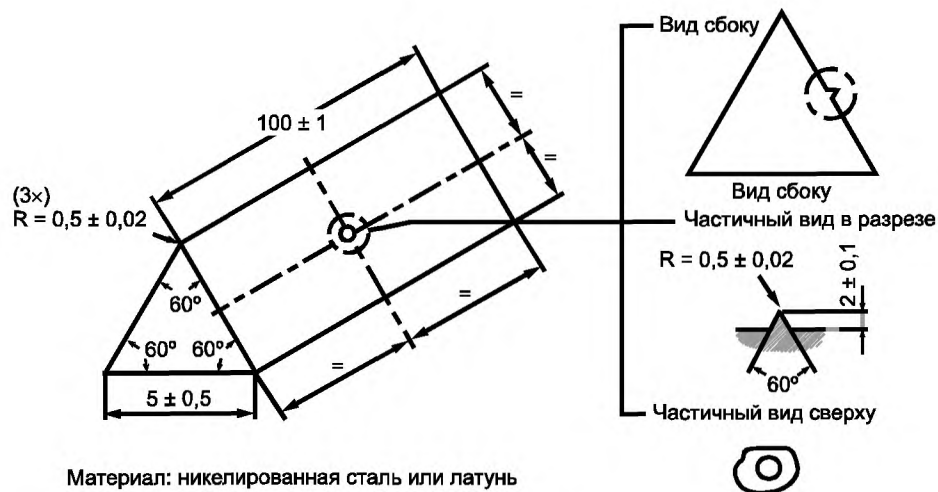
Рисунок 32 — Оправка
