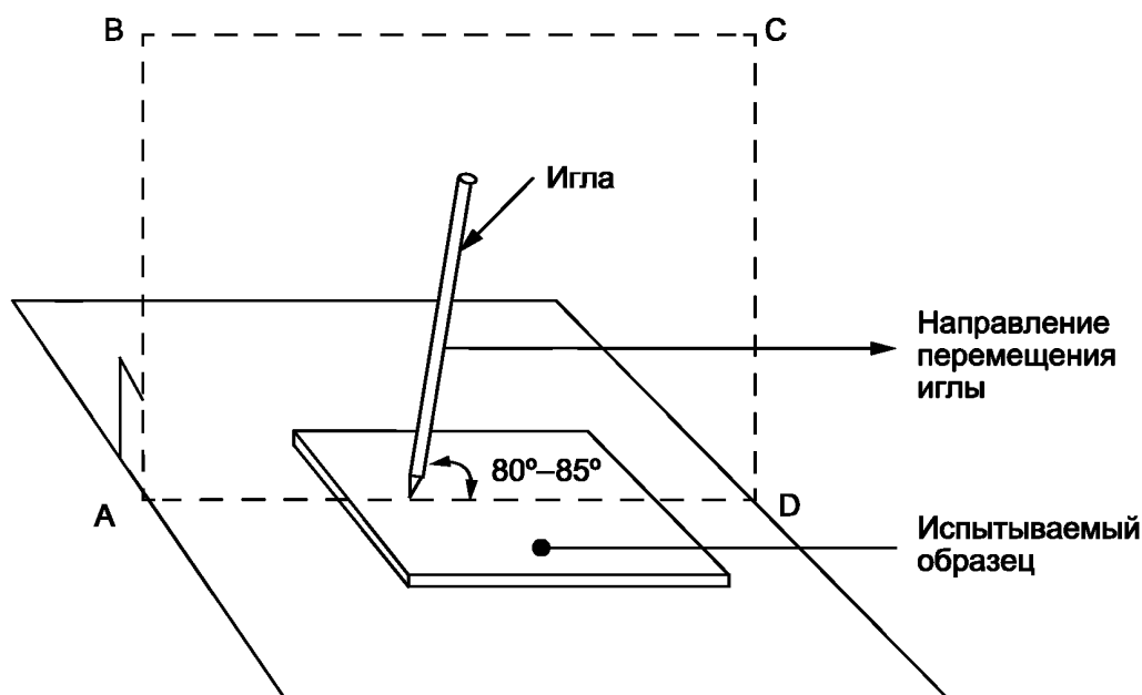
Рисунок G.3 — Испытание слоев покрытия на абразивную изнотостойчивость
