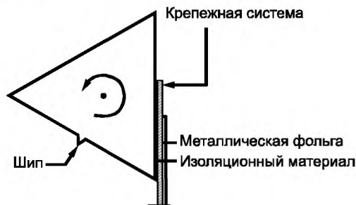
Рисунок 33 — Начальное положение оправки
