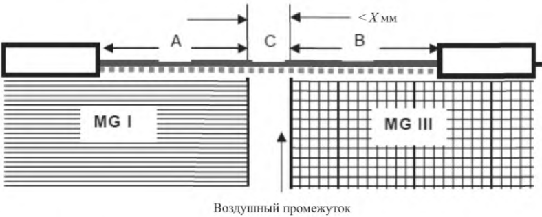
Рисунок О.17 — Материалы с разными значениями СИТ
