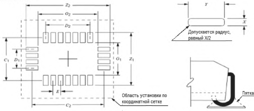
Рисунок 8 – Размеры посадочного места прямоугольного компонента QFJ, лист 1
