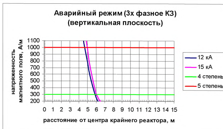
Рис.В.9 Распределение НМП при аварийных режимах в вертикальной плоскости при Z=0,25 \text{ Ом} ; n=34 ; R=0,6\text{м} ; S=2,4\text{м}
