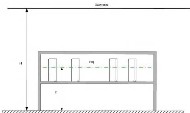
Рис.В.33 Расположение ошиновки над зданием РЦ
