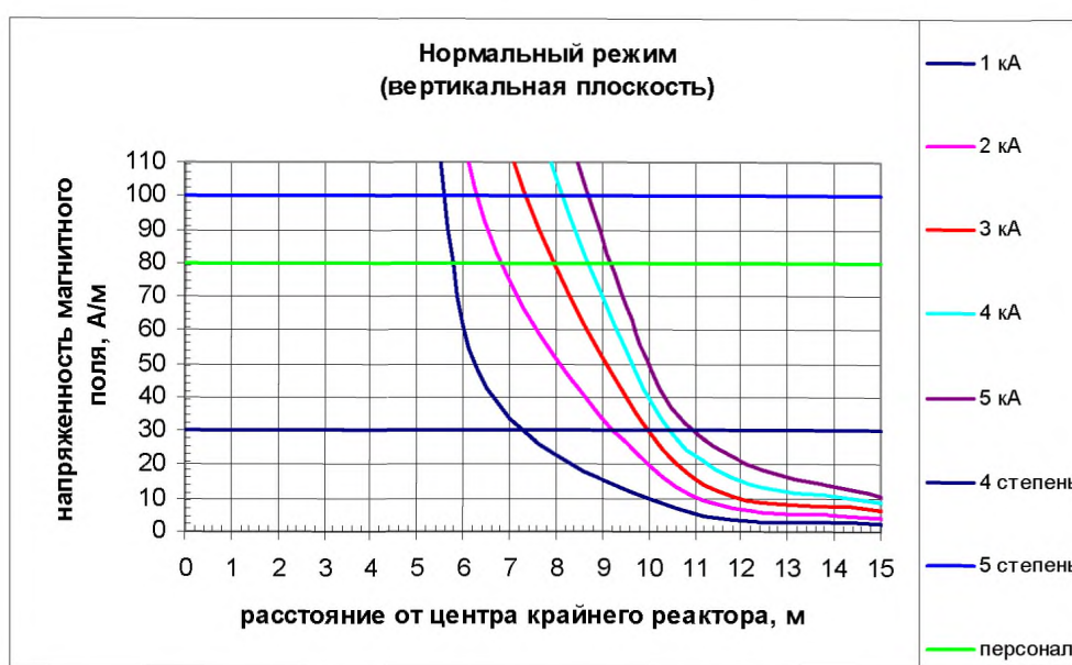
Рис.В.10 Распределение НМП при нормальных режимах в вертикальной плоскости при Z=0,96 \text{ Ом} ; n=45 ; R=0,9\text{м} ; S=2,4\text{м}
