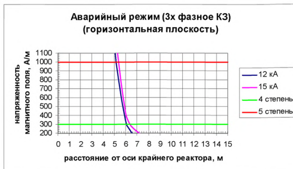
Рис.В.21 Распределение НМП при аварийных режимах в горизонтальной плоскости при Z=0,96 \text{ Ом} ; n=45 ; R=0,9\text{м} ; S=2,4\text{м}
