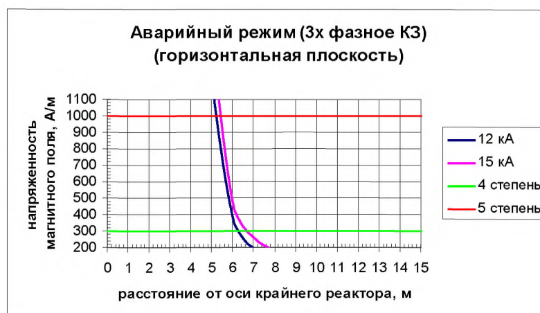
Рис.В.11 Распределение НМП при аварийных режимах в горизонтальной плоскости при ( Z=0,96 \text{ Ом} ; n=45 ; R=0,9\text{м} ; S=2,4\text{м} )
