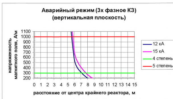
Рис.В.22 Распределение НМП при аварийных режимах в вертикальной плоскости при Z=0,96 \text{ Ом} ; n=45 ; R=0,9\text{м} ; S=2,4\text{м}
