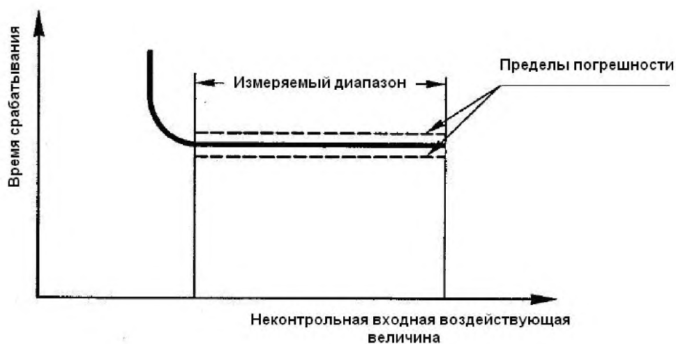
Рисунок 6 — Время срабатывания для реле мощности с независимой временной характеристикой
