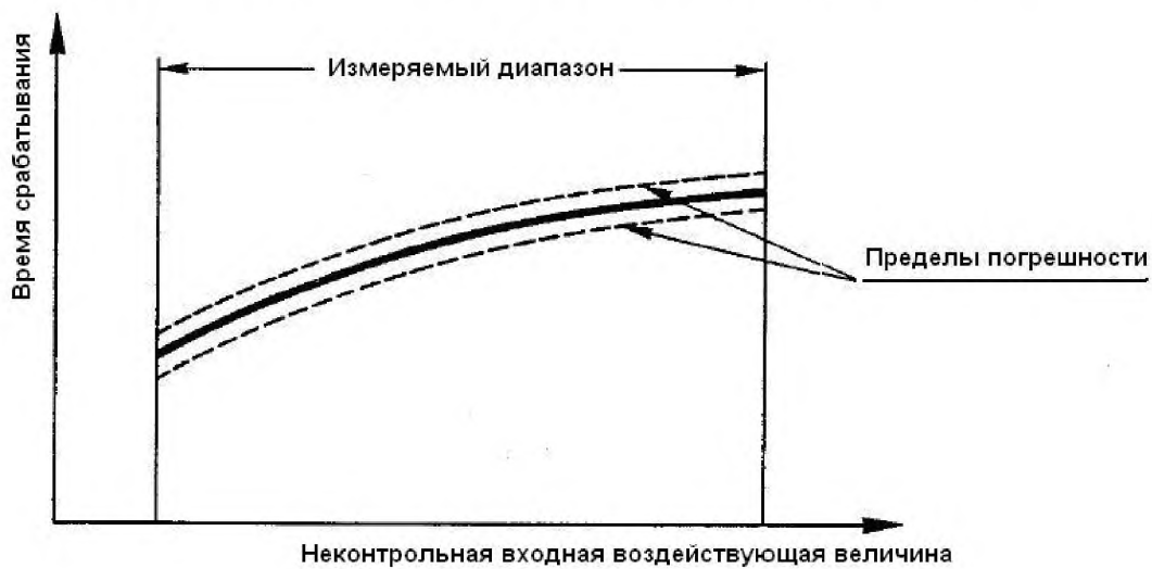
Рисунок 8 — Время срабатывания для реле направления с нормируемым временем
