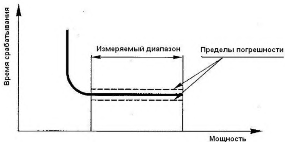
Рисунок 7 — Время срабатывания для реле направления с нормируемым временем
