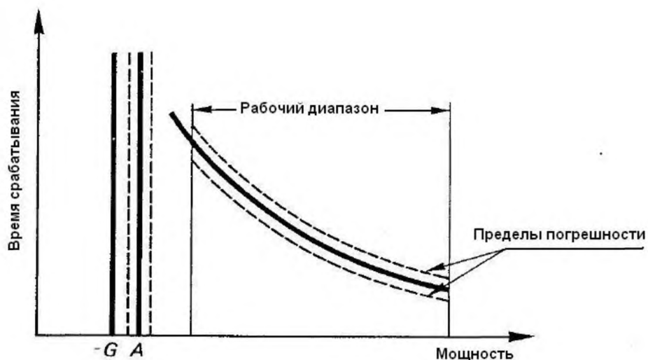
Рисунок 4 — Характеристика срабатывания реле направления с переменными значениями контрольной входной воздействующей величины
