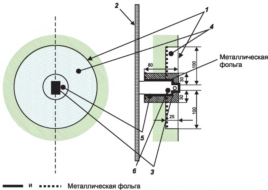
Размеры в миллиметрах. 1 – область основания, ограниченная поверхностью органа управления; 2 – монтажная панель; 3 – нажимная кнопка; 4 – область с задней поверхностью для защиты руки; 5 – область для защиты пальца; 6 – гнездо выключателя Рисунок R.2 – Оперативное пространство для нажимной кнопки
