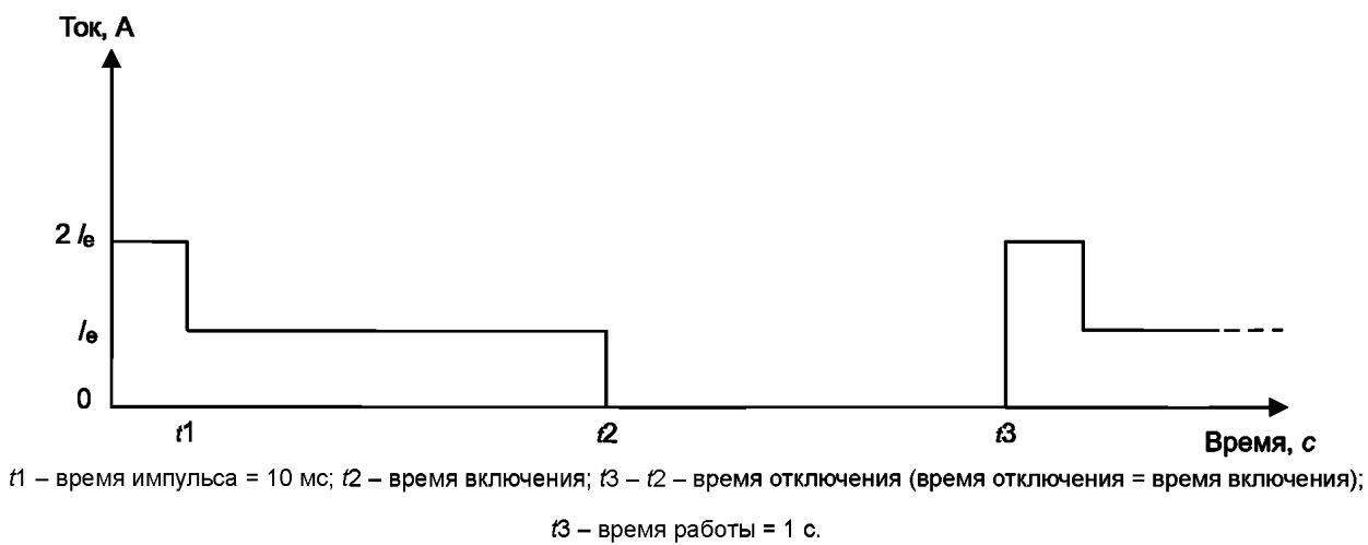
Рисунок S.4 – Временные интервалы коммутационного переключения для цифровых выходов постоянного тока
