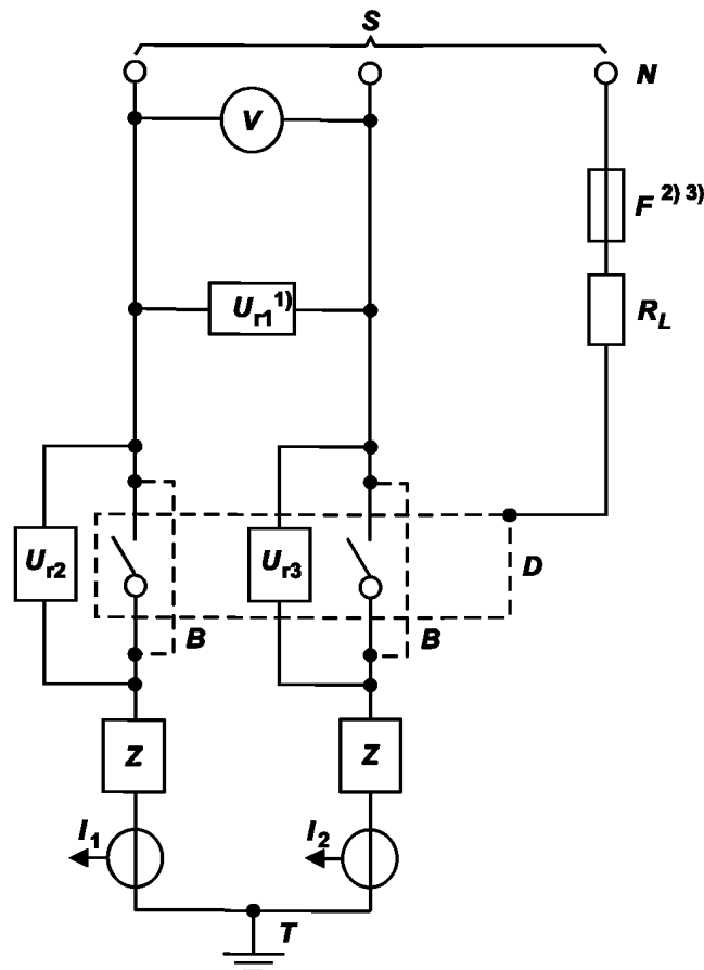
S – источник питания; U_{r1}, U_{r2}, U_{r3} – датчики напряжения; V – вольтметр; N – нейтраль (искусственная); F – плавкий элемент (8.3.3.5.2, перечисление g); Z – цепь нагрузки (см. рисунок 8); R_L – токоограничивающее сопротивление; D – испытуемый аппарат (с присоединенными проводниками); I_1, I_2 – датчики тока; B – переключки для настройки контура; T – точка заземления (на стороне нагрузки или питания).
