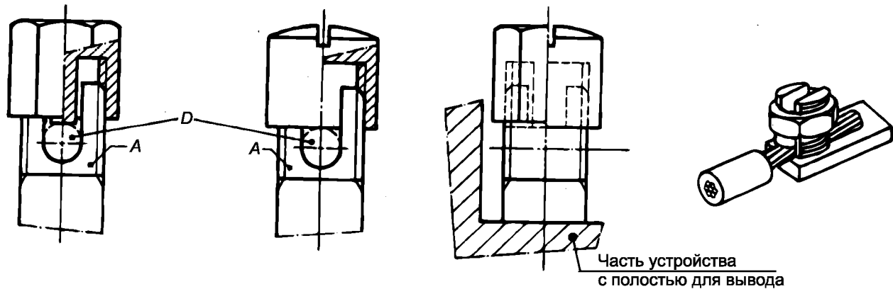
А – неподвижная часть; D – место для проводника. Зажим с крышкой – зажим резьбового типа, в котором проводник зажимается основанием прорези в резьбовом штифте с помощью гайки. Прижатие проводника осуществляется соответствующей формы шайбой под гайку или центральной шпилькой, если гайка колпачковая, или устройством равной эффективности, передающим давление от гайки проводнику внутри прорези Рисунок D.6 – Зажим с крышкой
