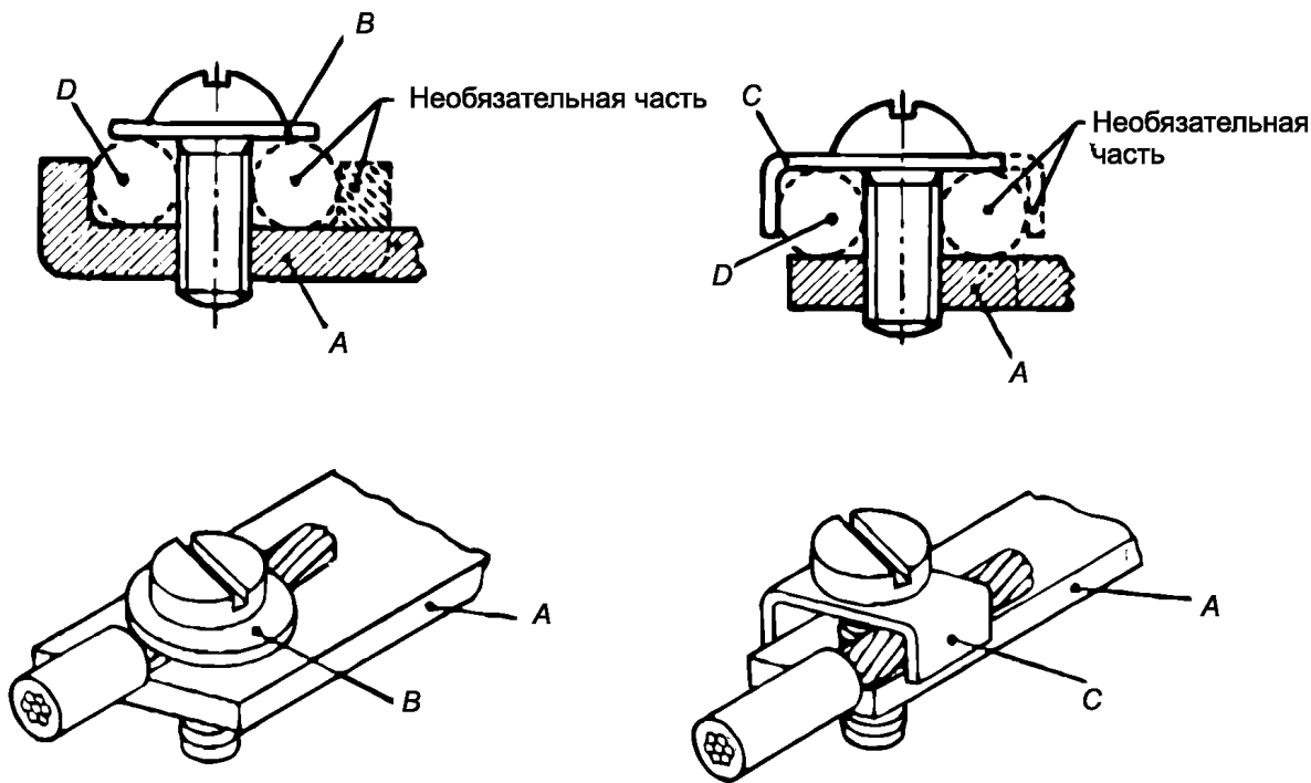
Выводы с прямым непосредственным давлением через головку винта
