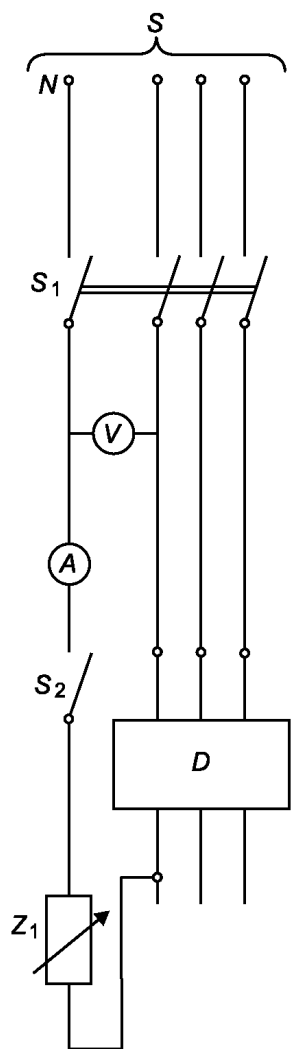
S – источник питания (трехфазный требуется только при необходимости питания аппарата); N – нейтраль; V – вольтметр; A – амперметр; S_1 – многополюсный выключатель; S_2 – однополюсный выключатель; D – испытуемое реле перегрузки; Z – регулируемое полное сопротивление.
