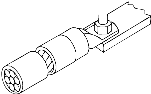
А – запорное устройство; В – кабельный наконечник или шина; F – неподвижная часть; Е – штифт Зажим под наконечник – резьбовой или штифтовой зажим предназначен для зажима кабельного наконечника или шины с помощью винта или гайки.
