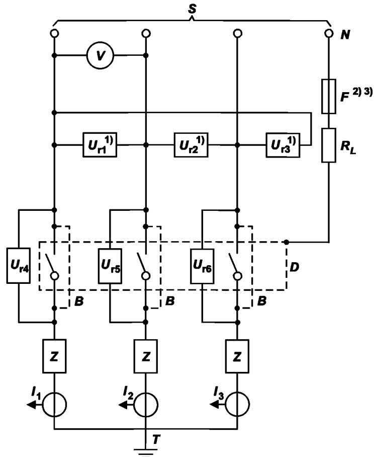
S – источник питания; U_{r1}, U_{r2}, U_{r3}, U_{r4}, U_{r5}, U_{r6} – датчики напряжения; V – вольтметр; N – нейтраль (искусственная); F – плавкий элемент (см. 8.3.3.5.2, перечисление g); B – переключки для настройки контура; Z – цепь нагрузки (см рисунок 8); R_L – токоограничивающие сопротивления; D – испытуемый аппарат (с присоединенными проводниками); I_1, I_2, I_3 – датчики тока; T – точка заземления (на стороне нагрузки или питания).
