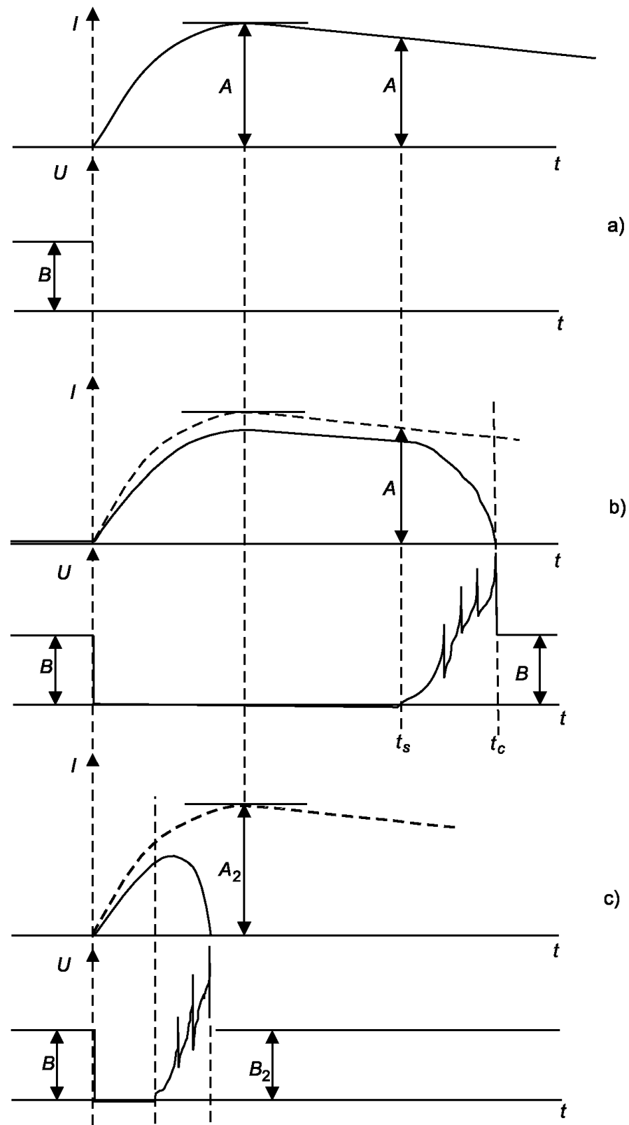
а) Калибровка цепи Ожидаемый пиковый ток включения A_2 б) Осциллограмма соответствующая отключению после того, как ток прошел свое максимальное значение Наибольшая отключающая способность: ток I = A при напряжении U = B_1 . Наибольшая включающая способность: ток I = A_2 при напряжении U = B . в) Осциллограмма, соответствующая отключению до того, как ток достигнет своего максимального значения Наибольшая отключающая способность: ток I = A_2 при напряжении U = B_2 . Наибольшая включающая способность: ток I = A_2 при напряжении U = B Рисунок 14 – Проверка наибольшей включающей и отключающей способностей при постоянном токе (см. 8.3.4.1.8)
