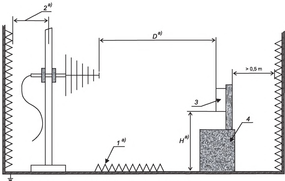
Рисунок 19 – Испытательная установка для проверки на устойчивость к излучаемым радиочастотным электромагнитным полям
