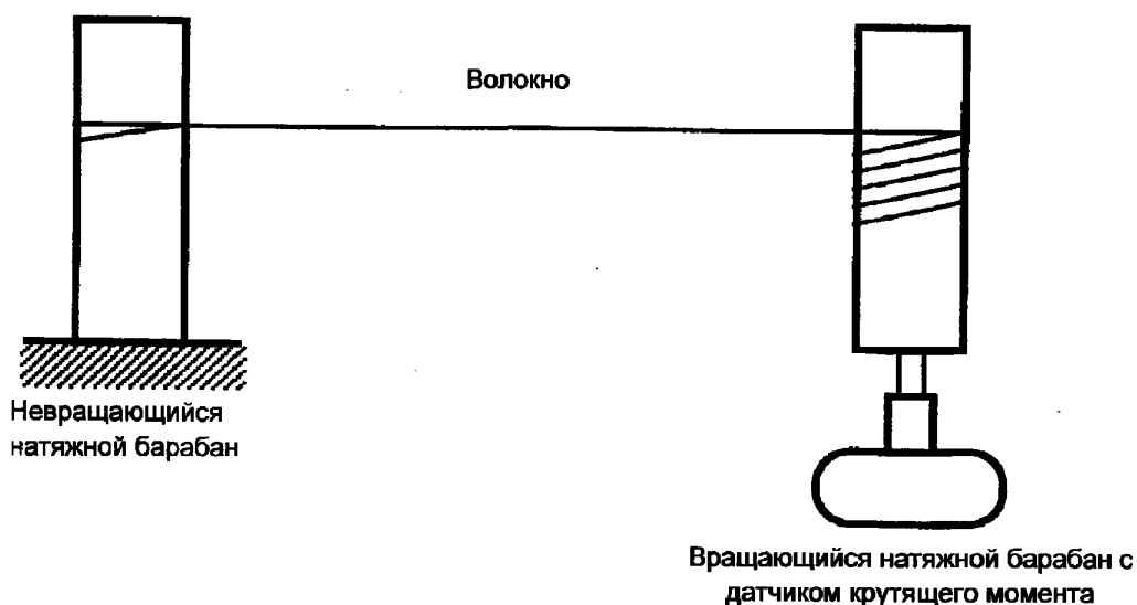
Рисунок А.2 — Схема ротационного испытательного оборудования
