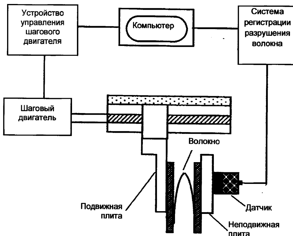
Рисунок В.1 — Схема установки двухточечного изгиба
