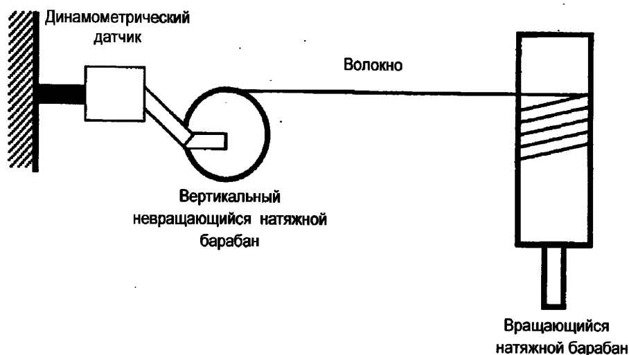
Рисунок А.2 — Схема ротационного испытательного оборудования
