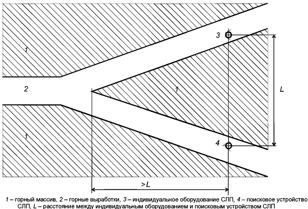
Рисунок В.1 — Схема проведения испытаний
