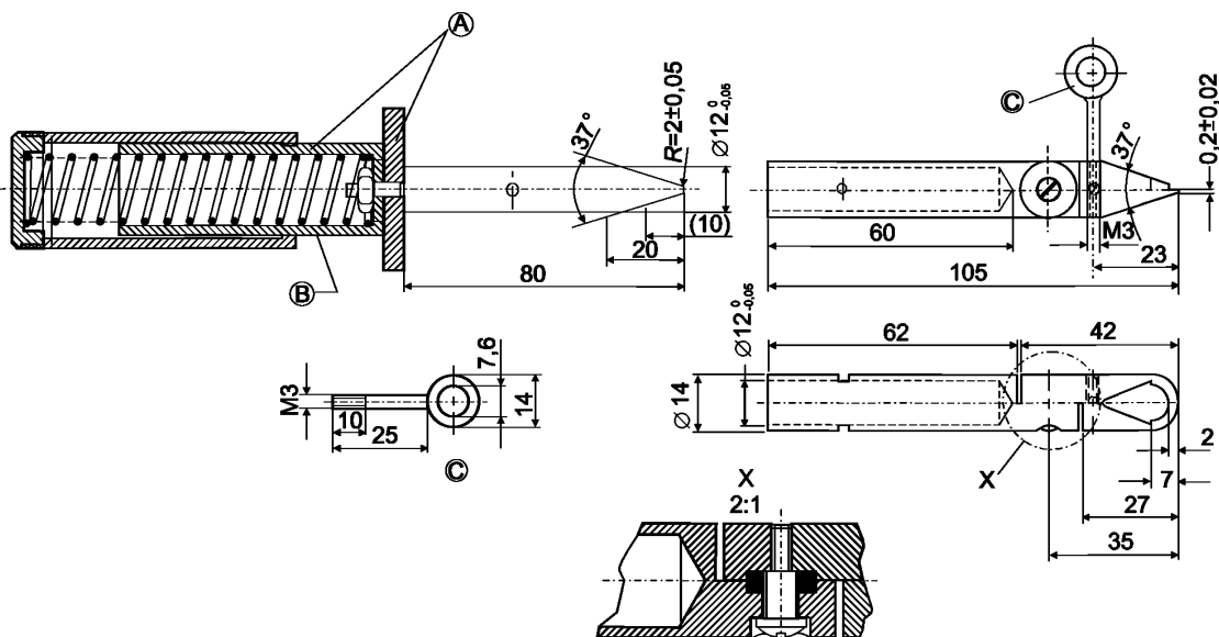
А — изоляционный материал; В — диаметр пружины; С — проушина Рисунок 1 — Испытательный ноготь
