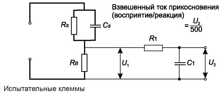
Рисунок С.3 — Цепь для измерения тока утечки
