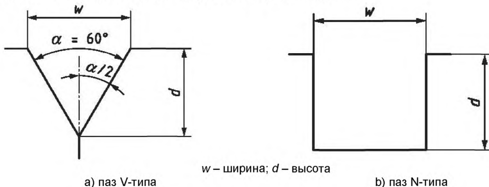
Рисунок 1 – Типы пазов
