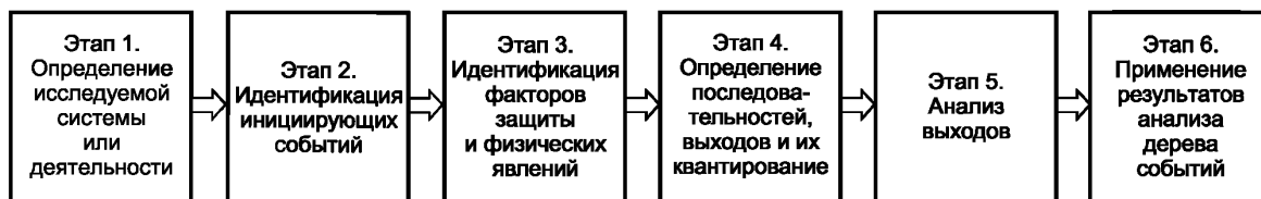
Рисунок 1 — Процесс разработки дерева событий
