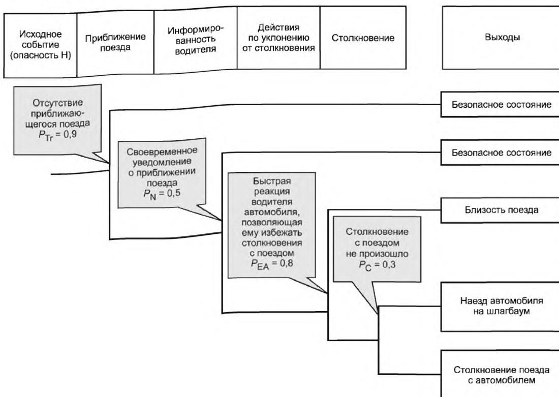
Рисунок В.4 — ЕТА для железнодорожного переезда
