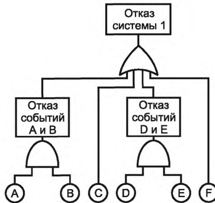
Рисунок В.6 — Дерево неисправностей для системы 1
