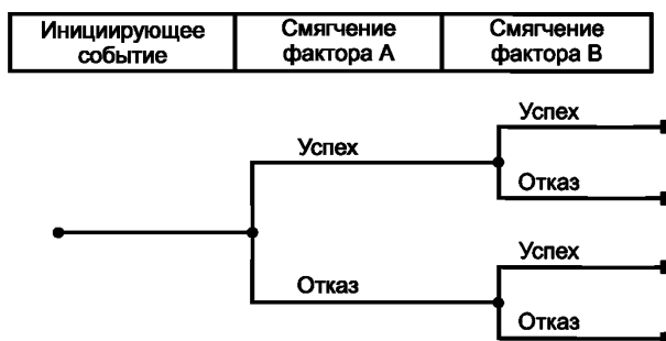
Рисунок 2 — Основное графическое представление дерева событий
