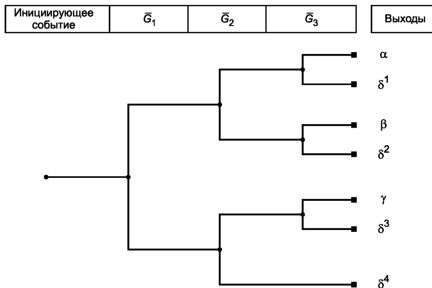
Рисунок В.9 — Дерево событий после «группировки отказов»
