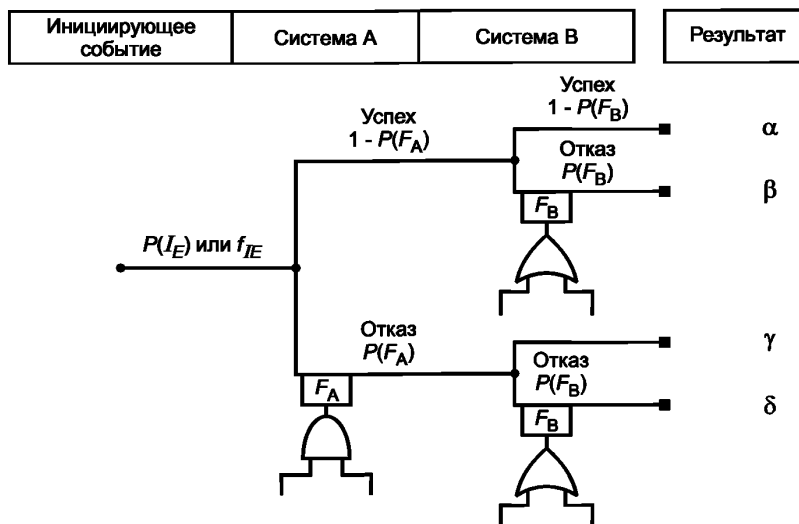
Рисунок 6 — Соединение с деревом неисправностей
