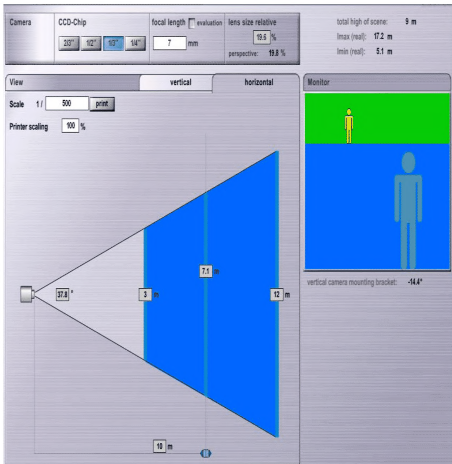
Рис. 2.5 Расчеты в программе ViewDesigner для камер БК-3, БК-6, БК-13, БК-14
