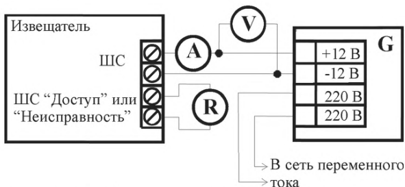
Рисунок 7.2 – Схема подключения извещателя формирующего извещения изменением тока потребления
