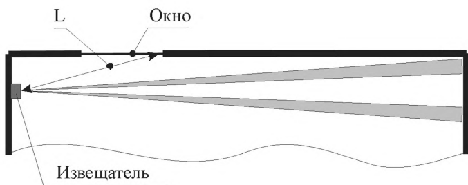
Рисунок 6.3 – Установка совмещенного извещателя с поверхностной ЗО ИК канала
