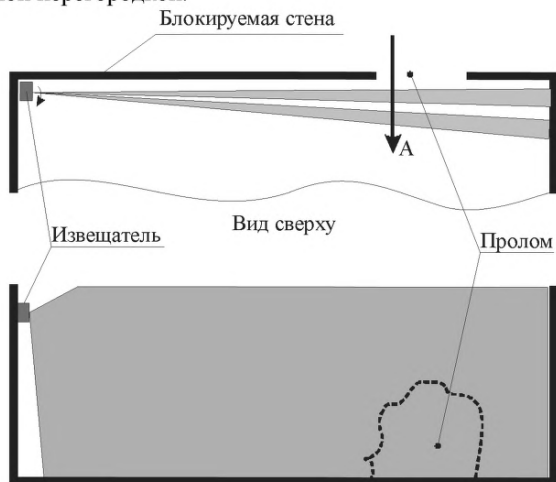
Рисунок 5.24 – Применение поверхностных извещателей для обнаружения проникновения через пролом в стене
