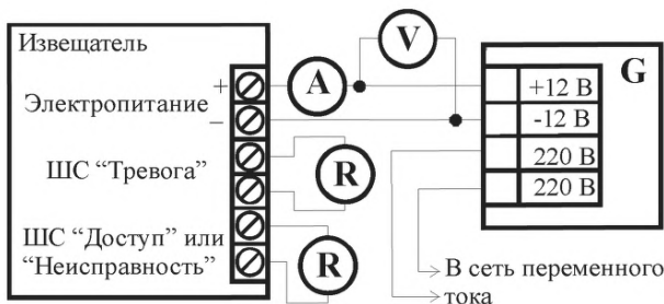
Рисунок 7.1 – Схема подключения извещателя формирующего извещения размыканием контактов реле (электронного ключа)
