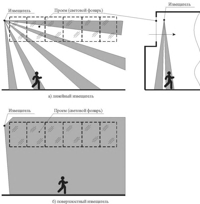
Рисунок 5.19 – Особенности применения извещателя, установленного на большой высоте
