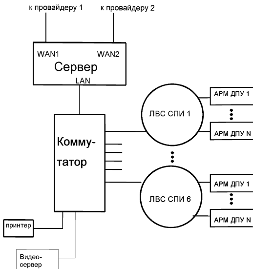
Рис. 7.1.2. Структура ЛВС ПЦО.
