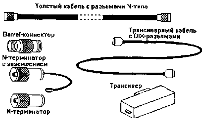
Рис. А.1.1. Аппаратура 10BASE5
