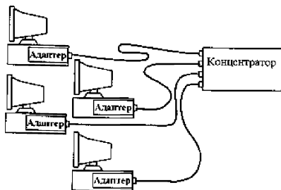
Рис. А.5.1. Схема объединения компьютеров по стандарту 100BASE-TX
