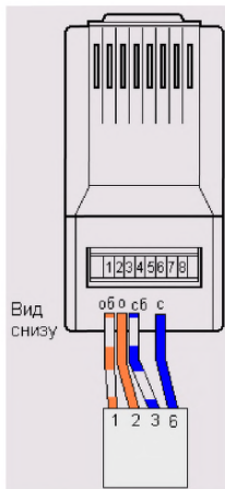
Рис. Б.13.2. Схема заделки четырехжильного кабеля «витая пара»
