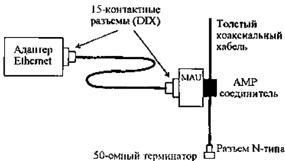
Рис. А.1.2. Подсоединение адаптера к толстому кабелю
