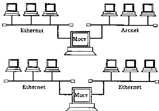
Рис. 5.1.1.4. Включение моста
