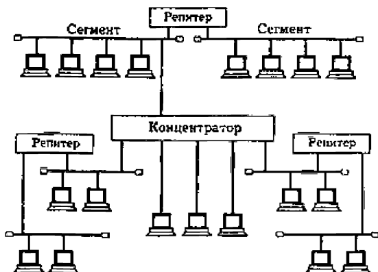
Рис. 5.2.1. Топология сети Ethernet
