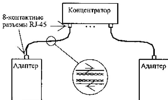
Рис. А.3.1. Подключения абонентов сети с помощью витой пары
