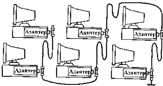
Рис. А.2.3. Соединение компьютеров сети тонким кабелем
