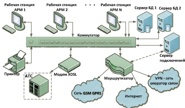
Рис. 6.3 Примерная схема организации на ПЦО локальной сети с основным и резервным сервером БД и сервером подключений (для СПИ «Приток-А»)
