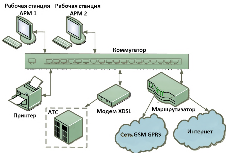
Рис. 6.1 Примерная схема организации одноранговой ЛВС на ПЦО
