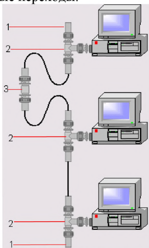
Рис. Б.3.1. Общая схема подключений в сети 10Base2
