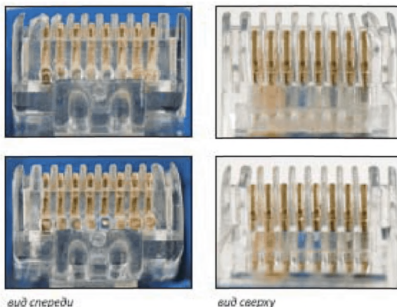
Рисунок 5: Для примера повреждений вилки RJ45, обнаруженных при поиске сбоя.
