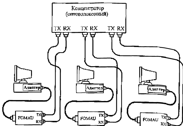
Рис. А.7.1. Подключение компьютеров к сети 100BASE-FX
