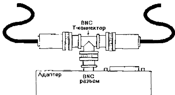
Рис. А.2.2. Присоединение адаптера к тонкому коаксиальному кабелю
