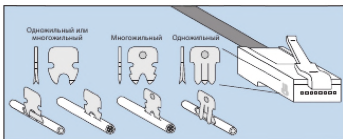
Рисунок 8.3.2.1 Виды зубцов в вилке RJ45 для многожильного (stranded) и одножильного (solid) кабеля.
