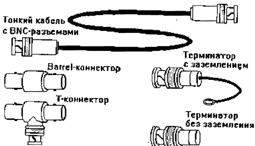
Рис. А.2.1. Аппаратура 10BASE2
