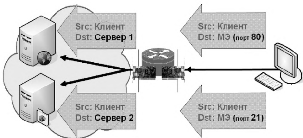
Рисунок 7.6.6.2. Технология векторизации адресов
