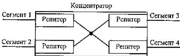
Рис. 5.1.1.3. Структура репитерного концентратора
