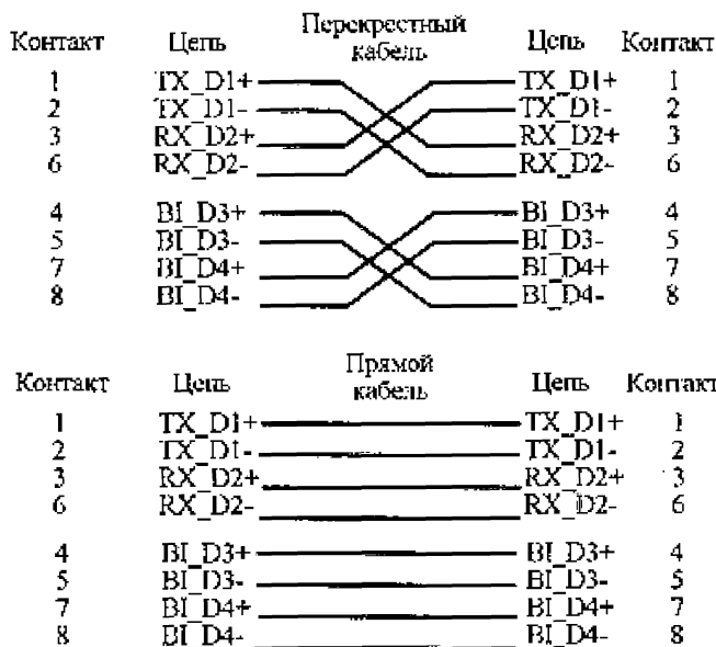
Рис. А.6.1. Прямой и перекрестный кабель сети 100BASE-T4
