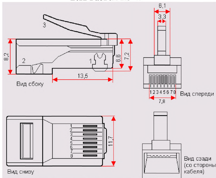
Рис. Б.12.1. Разъем RJ-45: 1 — контакты; 2 — держатель кабеля; 3 — замок разъема
