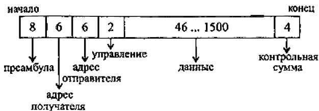
Рис. 5.2.2. Структура пакета сети Ethernet, (цифры показывают количество байт)
