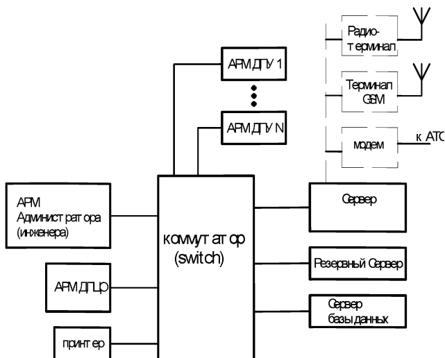
Рис. 7.1.1. Структура ЛВС СПИ.
