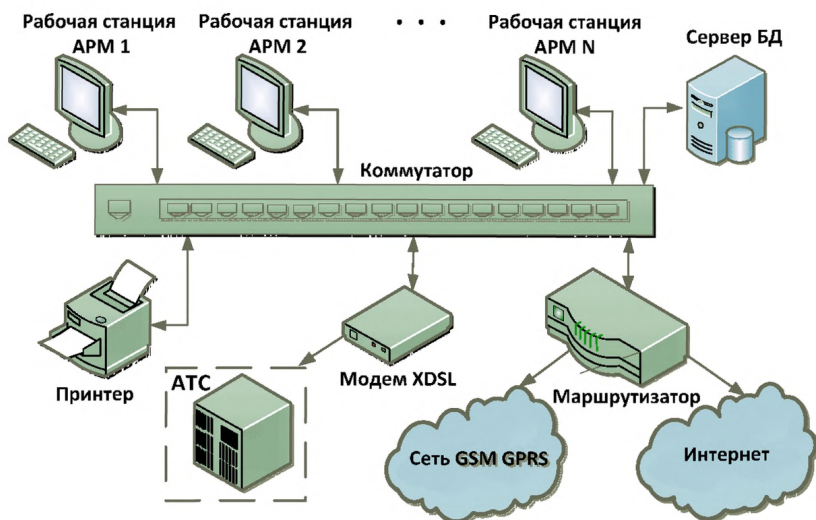
Рис. 6.2 Примерная схема организации на ПЦО локальной сети с сервером БД
