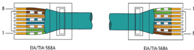
Рис. Б.13.1.а) Нумерация контактов в разъеме.
