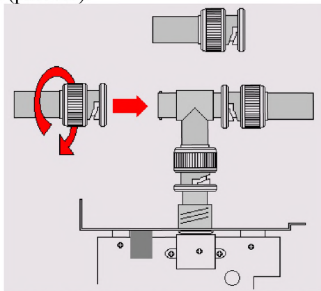
Рис. Б.5.1. Установка терминатора
