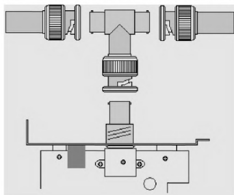
Рис. Б.4.1. Т-коннектор
