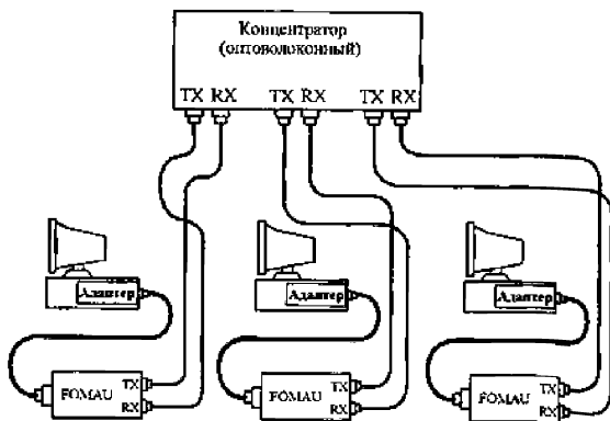
Рис. А.4.4. Объединение компьютеров в сеть по стандарту 10BASE-FL
