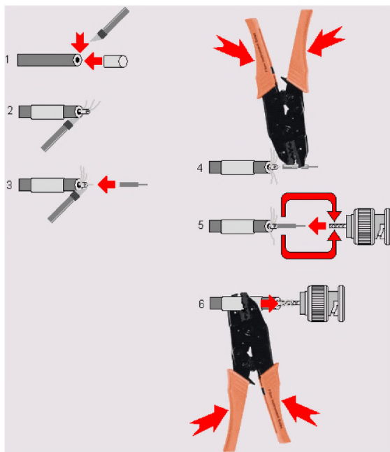
Рис. Б.2.3. Порядок монтажа разъема BNC
