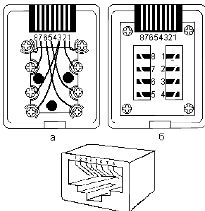
Рис. Б.14.1. Сетевая розетка RJ-45
