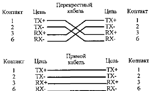
Рис. А.3.3. Соединение проводов прямого и перекрестного кабелей сегмента 10BASE-T
