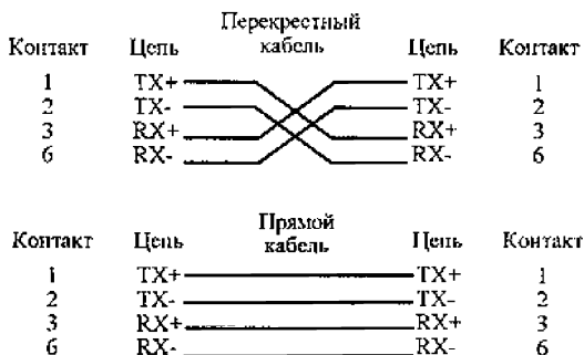
Рис. А.5.3. Прямой и перекрестный кабели, применяемые в сегменте 100BASE-TX
