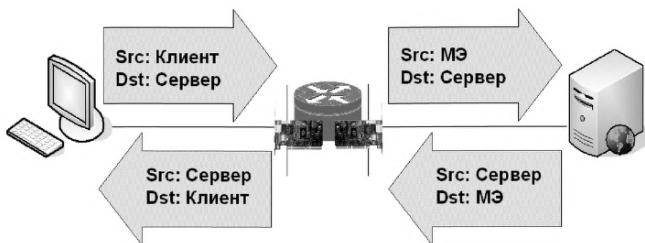
Рисунок 7.6.6.1. Технология NAT
