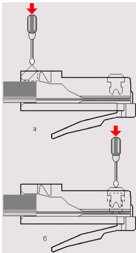
Рис. Б.15.1. Монтаж разъема RJ-45 без обжимного инструмента
