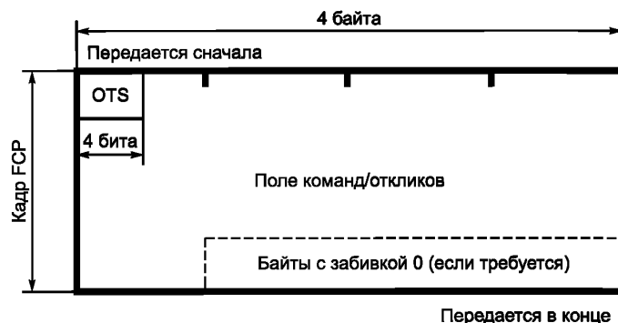
Рисунок 32 — Структура кадра FCP
