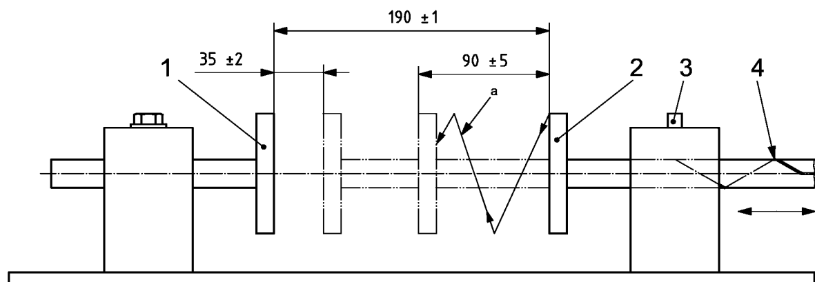
а) Движение диска
