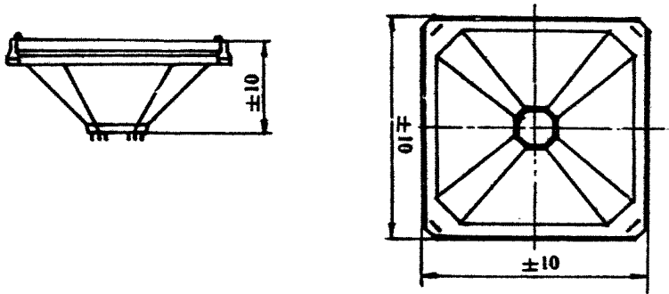
Рис.3. Воронки
