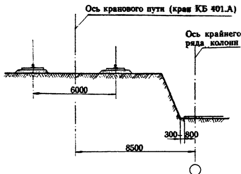
Рис.I.Схема привязки башенного крана КБ-40I.A к осям сооружения при бетонировании фундаментной плиты
