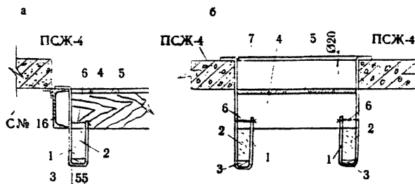
Рис.35. Опираие металлических крюков на металлические балки (а) и железобетонные плиты (б); 1 - металлические крюки; 2 - деревянный прогон 50х150 мм; 3 - клиновой злапы; 4-деревянная балка 50х150 мм; 5 - опалубочный настил из досок \delta = 25 мм; 6 - проволочная зкрутка; 7 - растерный металлический прут \phi 20 мм, соединенный на сварке с опорной частью крюков (1)
