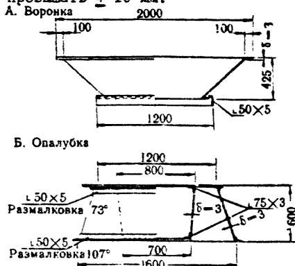
Рис.2. Металлическая опалубка и воронка для бетонирования подколонников
