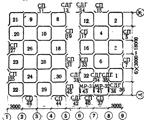
Рис.24.Схема последовательности монтажа элементов стен рабочего здания РЗС 4х175 (пример 5 ряда)
