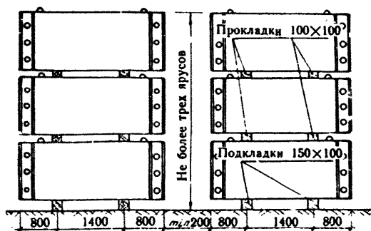
Рис.6. Правила складирования объемных стеновых элементов СВО
