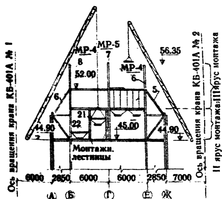
Рис. 33. Схема монтажа металлических бункеров на отметке 52.00 в надстройке рабочего здания РЗС 4х175
