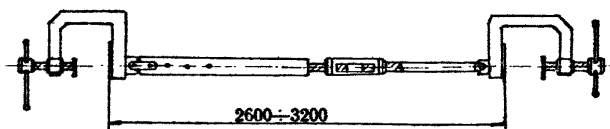
Рис.26. Универсальная струбина (ЦНИИОМТП)
