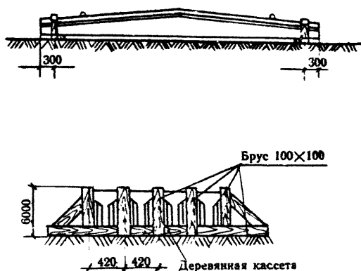
Рис.9. Правила складирования балок в деревянных кассетах.
