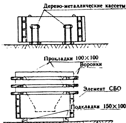
Рис.6. Правила складирования объемных стеновых элементов СВО
