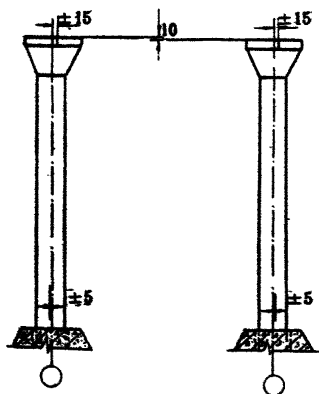
Рис.II. Допускаемые отклонения при монтаже колонн подсилоного этажа
