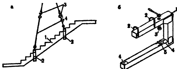
Рис.23. Монтаж лестничных маршей: а). Схема строповки марша: 1 - лестничный марш, 2 - вилочный подхват, 3 - крюки четырехветвевых стропов, 4 - удлинители; б). Вилочный подхват: 1-скоба, 2 - монтажные петли, 3 - прижимной винт, 4 - опоры, 5-упор
