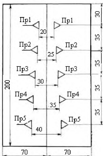
Рисунок 4 – Огнеупорная подставка с пироскопами
