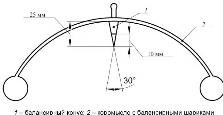
Рисунок 3 – Балансирный конус
