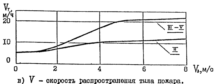
Рис. 4.1. Зависимость линейной скорости распространения низового пожара от скорости ветра ( V_{в} ) для насаждений I-го класса горимости (римскими цифрами обозначены классы пожарной опасности погоды).
