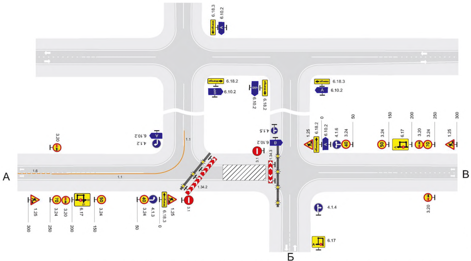
Рисунок Б.13 - Двухполосная дорога. Рабочая зона долговременных работ на всей ширине проезжей части. Пропуск транспортных средств по существующим дорогам
