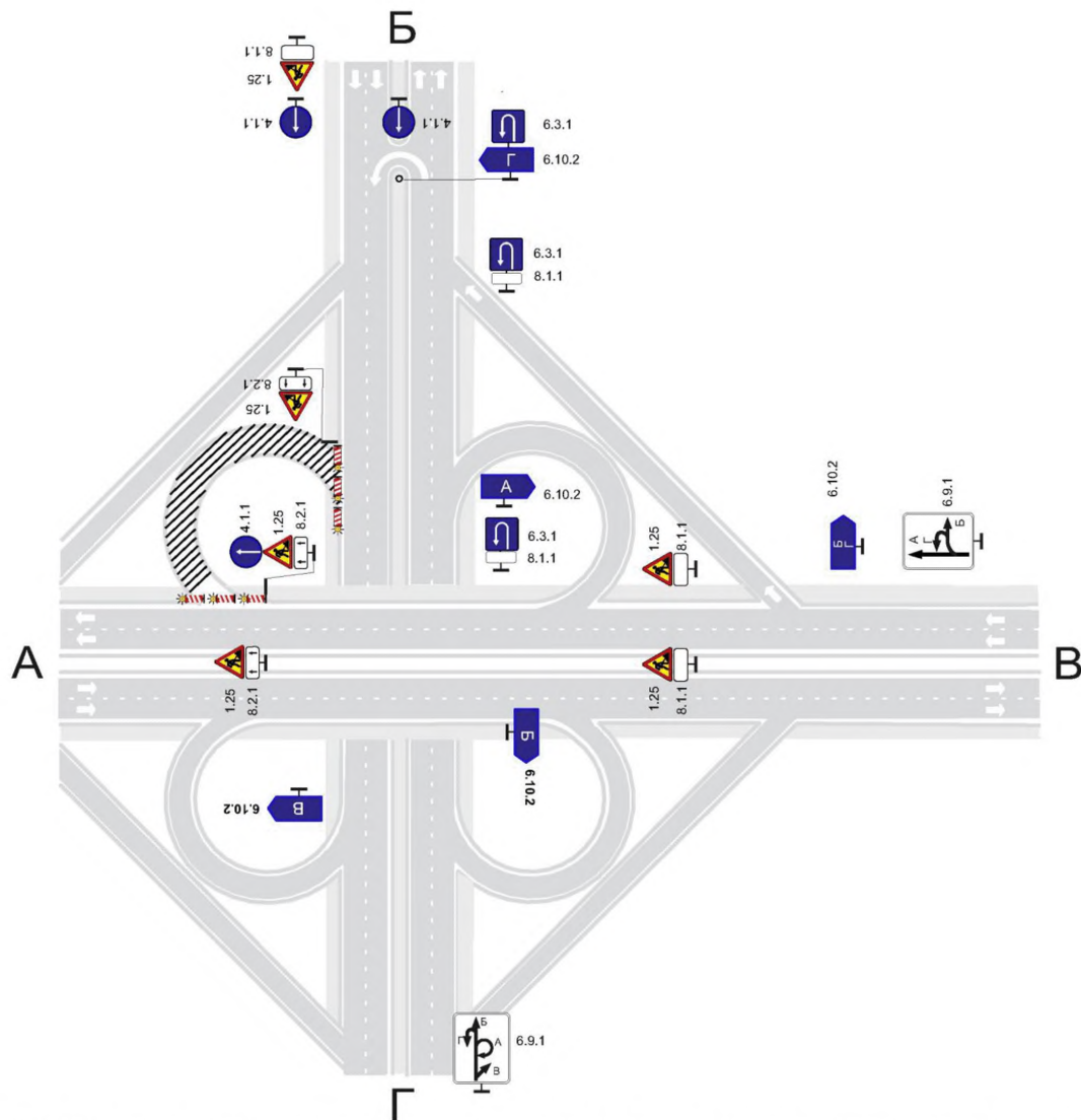
Рисунок Б.31 - Транспортная развязка - клеверный лист. Зона производства работ на левоворотном съезде. Пропуск транспортных средств по правоповоротному съезду с устройством разворота на одной из дорог
