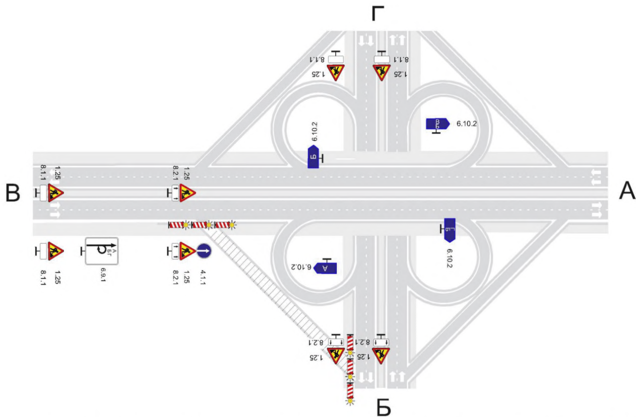
Рисунок Б.32 - Транспортная развязка - клеверный лист. Зона производства работ на правоповоротном съезде. Пропуск транспортных средств по левоповоротным съездам
