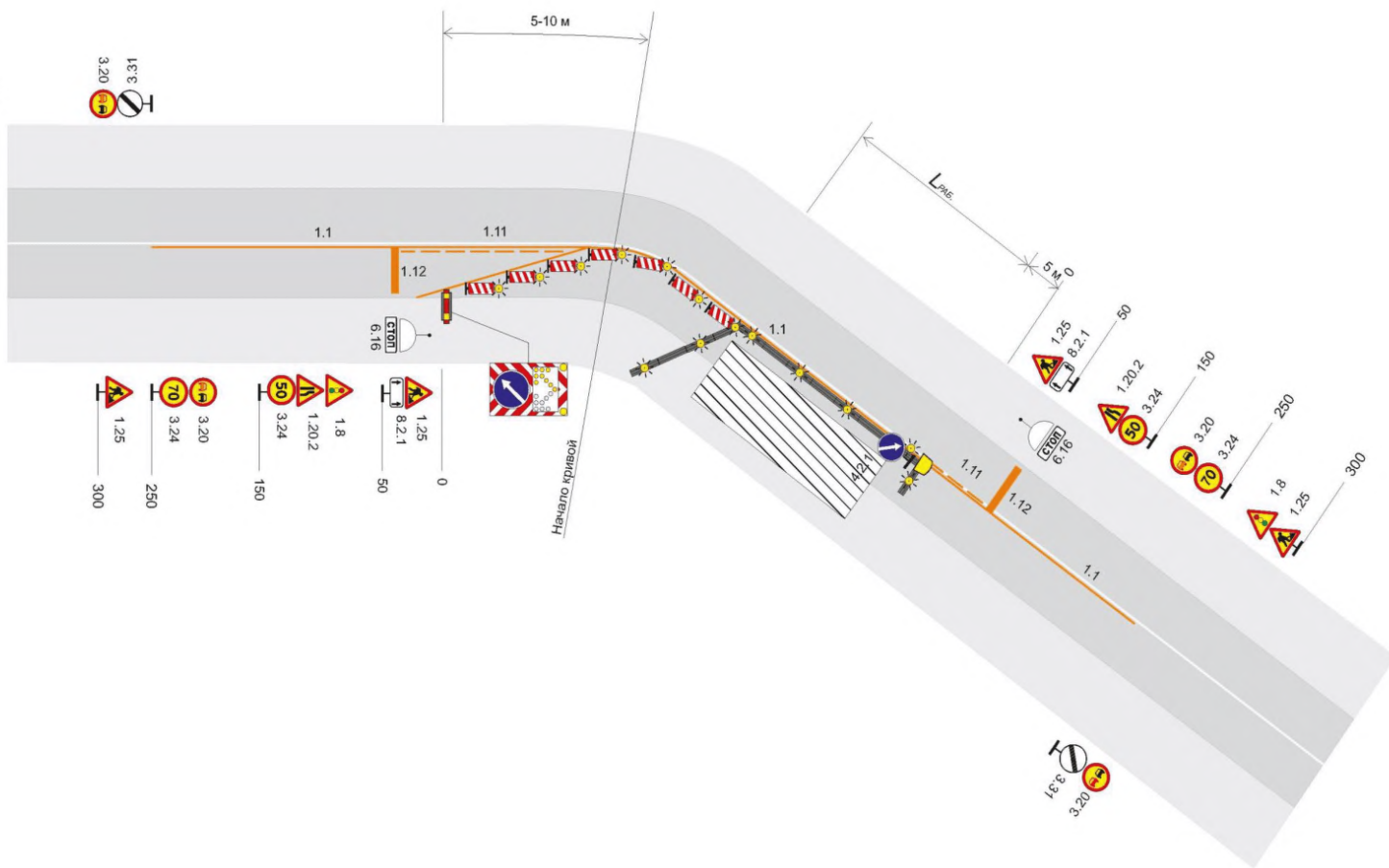
Рисунок Б.4 - Двухполосная дорога. Рабочая зона долговременных работ на полосе движения. Пропуск транспортных средств встречных направлений по одной полосе с помощью светофорного регулирования при ограниченной видимости
