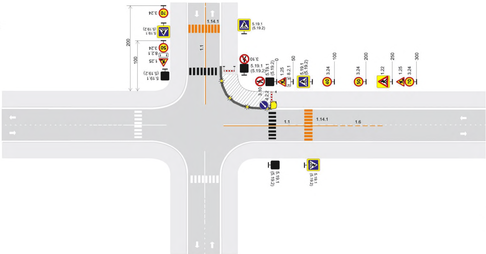
Рисунок Б.12 - Двухполосная дорога. Рабочая зона долговременных работ на пересечении в одном уровне на обочине
