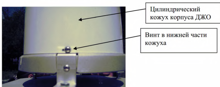
Рисунок 10.7 – Расположение винтов на корпусе ДЖО
