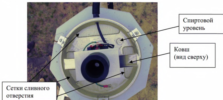
Рисунок 10.8 – Внутренняя конструкция ДЖО (вид сверху)
