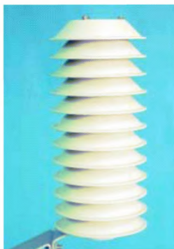
Рисунок 8.2 – Радиационная защита DTR 502 (а) и DTR 13 (б)
