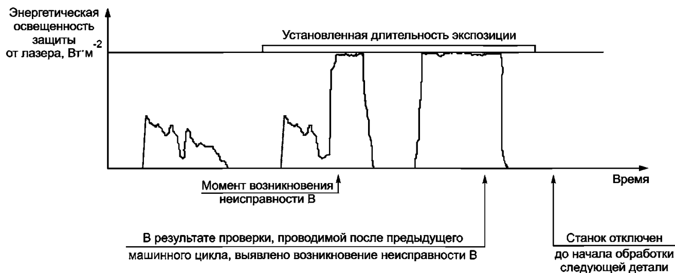
Рисунок В.6b — Отключение лазера при использовании автономного машинного мониторинга безопасности
