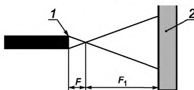
1 — линза; 2 — защита
