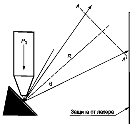
Рисунок В.2 — Расчет зеркального отражения
