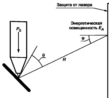
Рисунок В.1 — Расчет диффузного отражения
