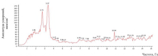
Рисунок В.6 – Спектр сигнала, приведенного на рисунке В.5
