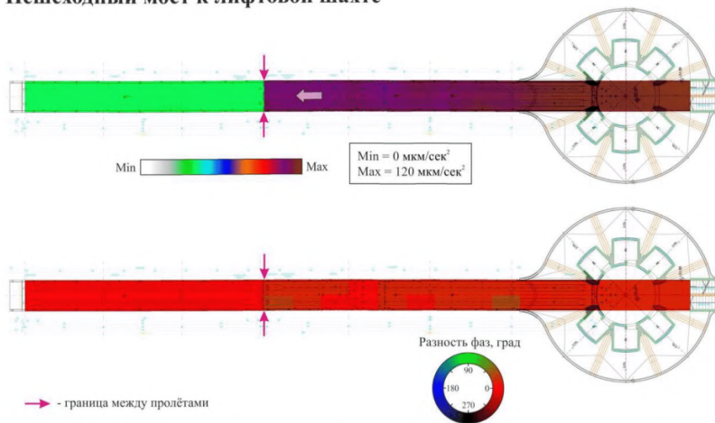
Рисунок В.12 – Пример карт амплитуд и фаз продольного колебания
