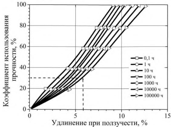
Рисунок 7.6 – Изохронные кривые ползучести
