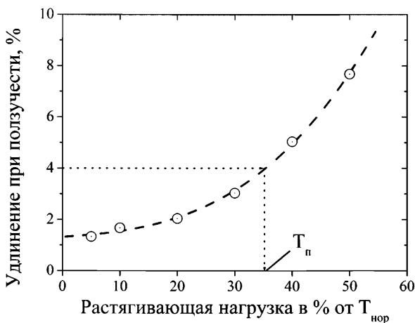
Рисунок 7.4 – Изохронная кривая «растягивающая нагрузка – относительное удлинение» при заданном времени t
