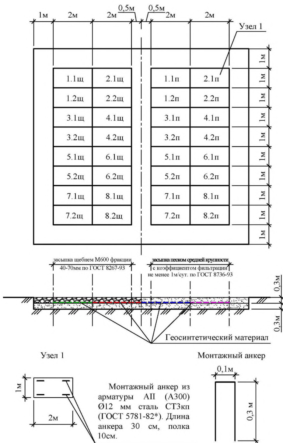
Рисунок 6.1 – Схема испытательного полигона
