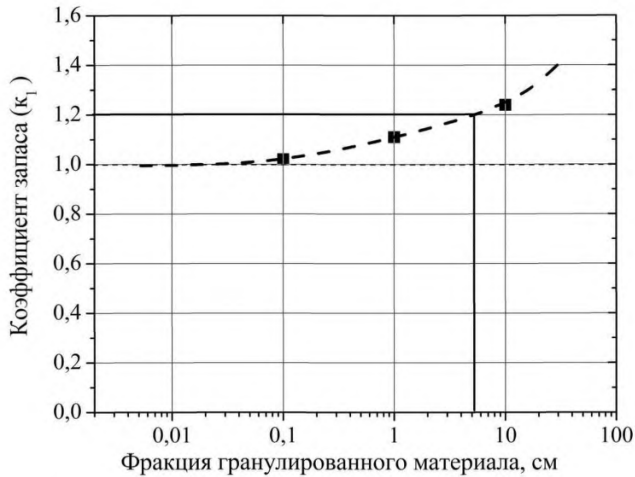
Рисунок 6.2 – Интерполяция коэффициента учета k_1
