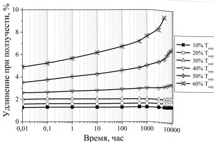
Рисунок 7.2 – Ползучесть геосинтетического материала при разных уровнях задаваемой нагрузки
