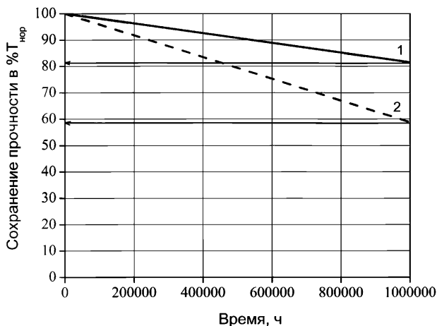
Рисунок 10.3 – Кривая старения при температуре эксплуатации
