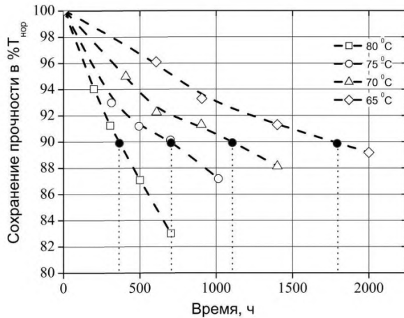
Рисунок 10.1 – Снижение прочности при заданных температурах
