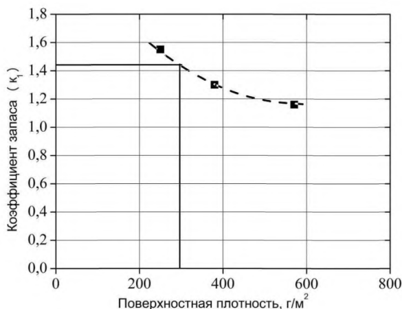
Рисунок 6.3 – Интерполяция k_1 от измерений повреждений на материалах одной серии, отличающихся только поверхностной плотностью
