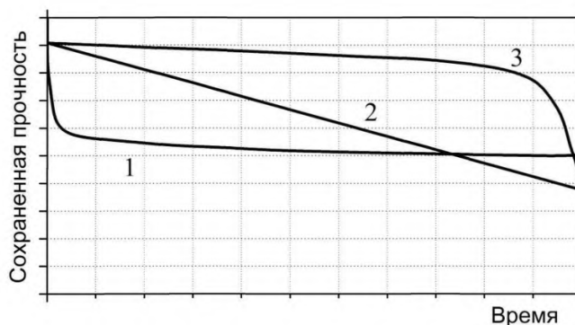
Рисунок 5.3 – Сохраненная доступная прочность в зависимости от времени для трех режимов ухудшения свойств
