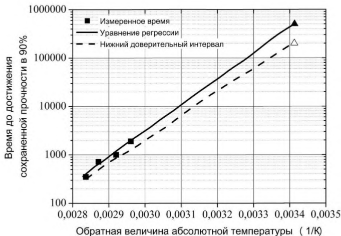
Рисунок 10.2 – Диаграмма Арениуса
