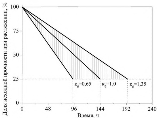
Рисунок 11.1 – Зависимость прочности при растяжении от времени контакта образцов с испытательным грунтом
