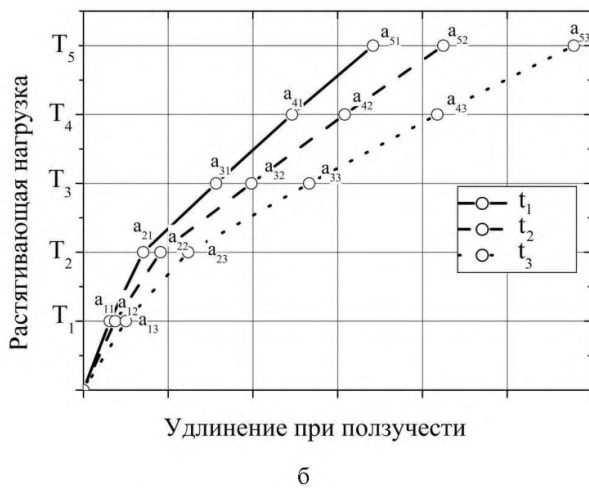
Рисунок 7.5 – Ползучесть геосинтетического материала (а) и изохронные кривые ползучести (б)
