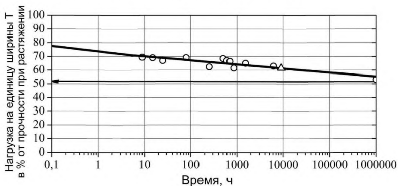
Рисунок 7.10 – Кривая длительной прочности при ползучести с линейной аппроксимацией
