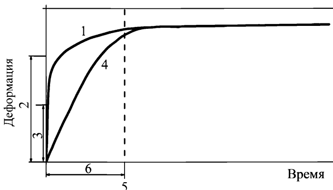
1 – испытание на ползучесть в лаборатории; 2 – деформация за период приложения нагрузки в конструкции; 3 – деформация за период приложения нагрузки при испытаниях на ползучесть; 4 – нагружение и ползучесть армирующего компонента в конструкции; 5 – новое время 0 ползучести после строительства; 6 – время строительства конструкции Рисунок 7.1 – Концептуальная иллюстрация для сравнения ползучести, измеренной в конструкции, с данными ползучести, полученными в лаборатории
