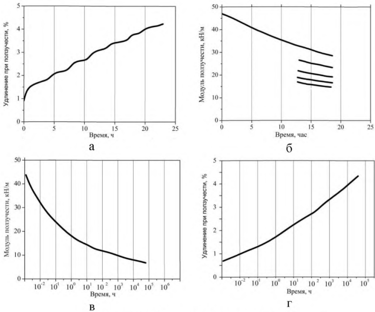
Рисунок 7.8 – Метод ступенчатых изотерм
