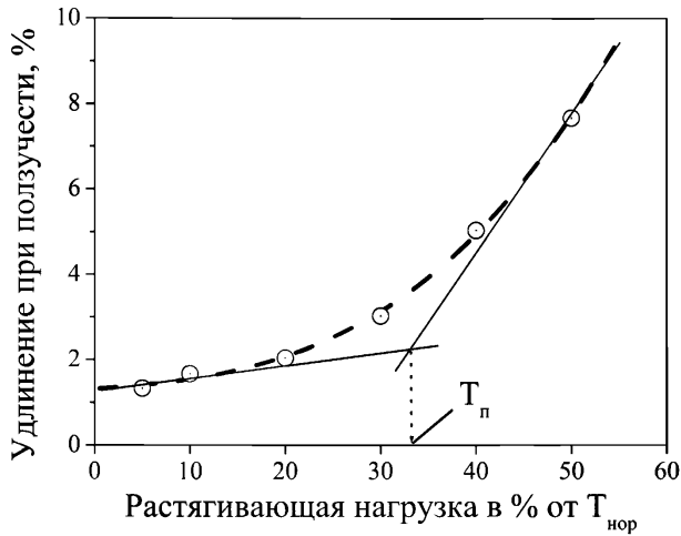
Рисунок 7.3 – Изохронная кривая «растягивающая нагрузка – относительное удлинение» при заданном времени t
