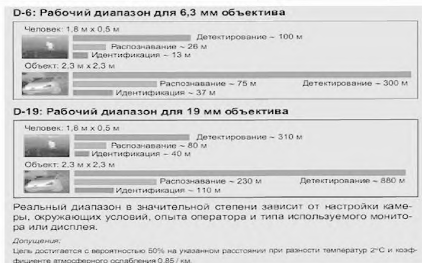
Рис. 129 Рабочий диапазон объективов камер серии D
