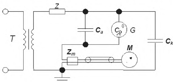
Рисунок В.3 – Пример симметричной испытательной схемы
