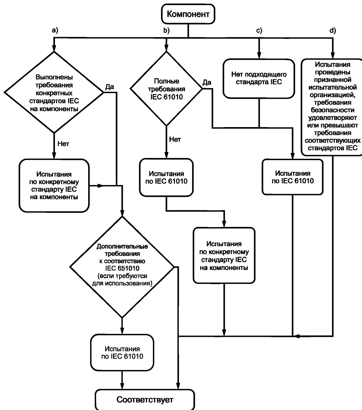
Рисунок 15 — Алгоритм вариантов проверки соответствия по 14.1, перечисления а), b), c) и d)
