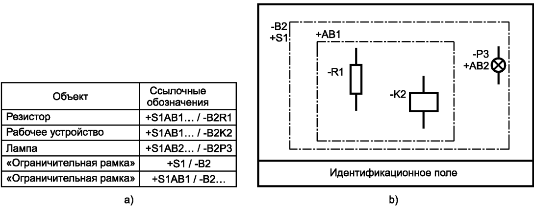
a) ссылочные обозначения объектов b) ссылочные объекты, показанные на схеме
