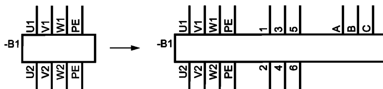
Рисунок 11 — Пример расширения символического обозначения
