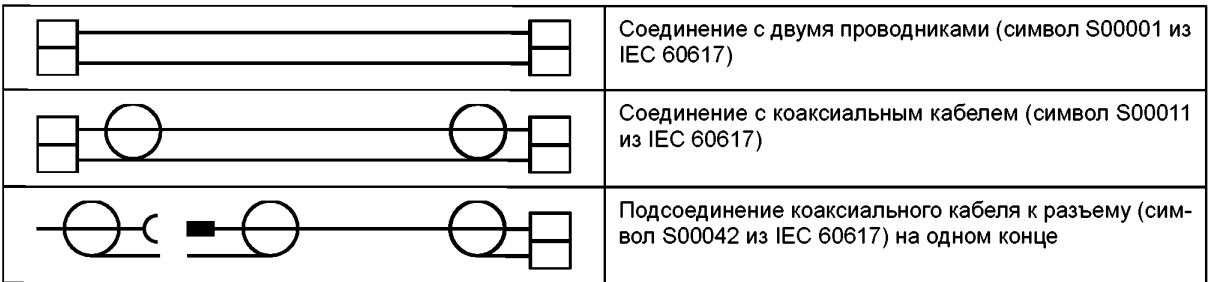
Рисунок 80 — Пример кабельных соединений
