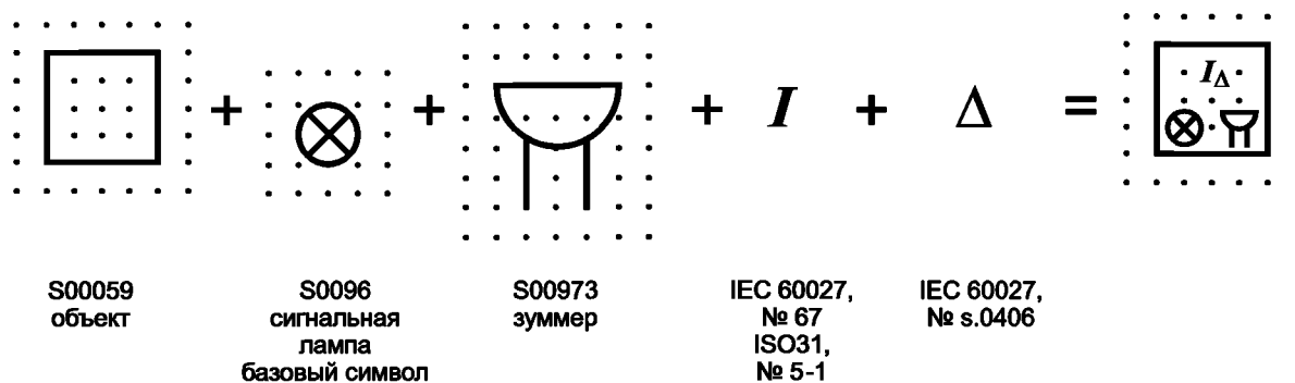
Рисунок А.11 — Пример символа для представления RCM
