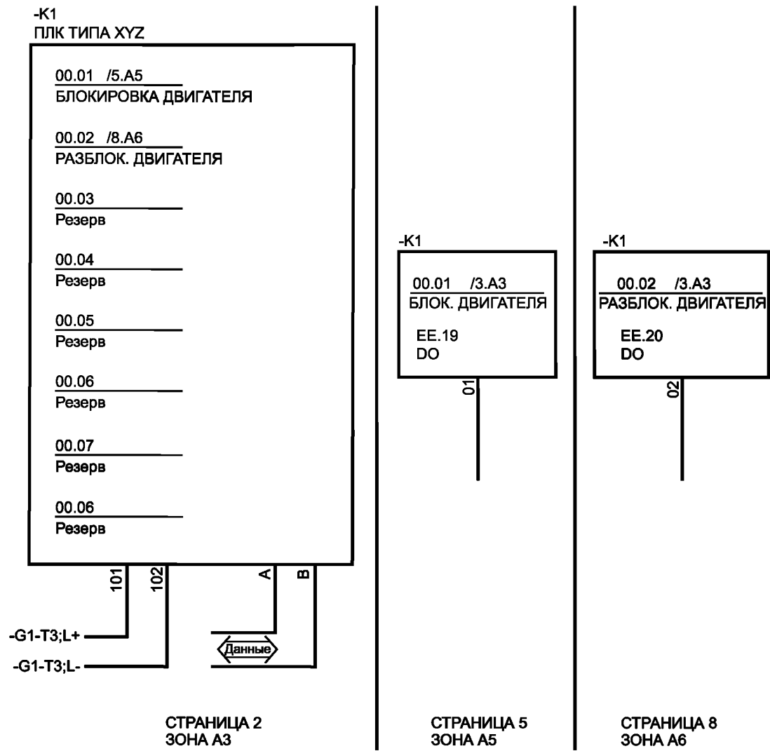
Рисунок А.12 — Символические представления для ПЛК
