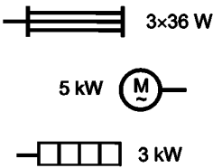
Рисунок 84 — Представление технических данных
