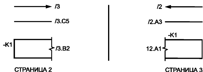
Рисунок 8 — Примеры использования перекрестных ссылок
