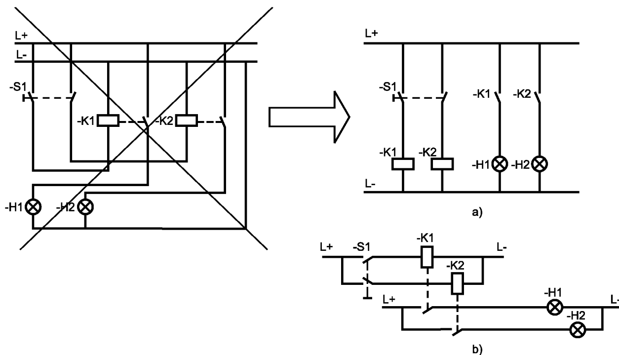
a) раздельное представление многосимвольного отображения компонентов b) частично соединенное представление многосимвольного отображения компонентов
