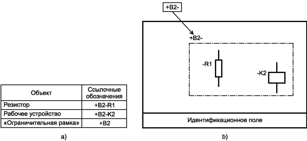
a) ссылочные обозначения объектов b) ссылочные объекты, показанные на схеме
