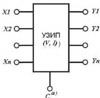
1f – многовыводное УЗИП
