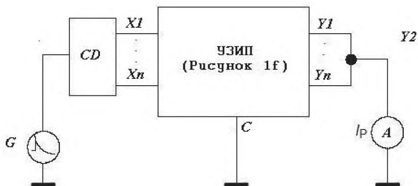
Рисунок Е.6 – Определение сквозного тока общего вида для многвыводных УЗИП
