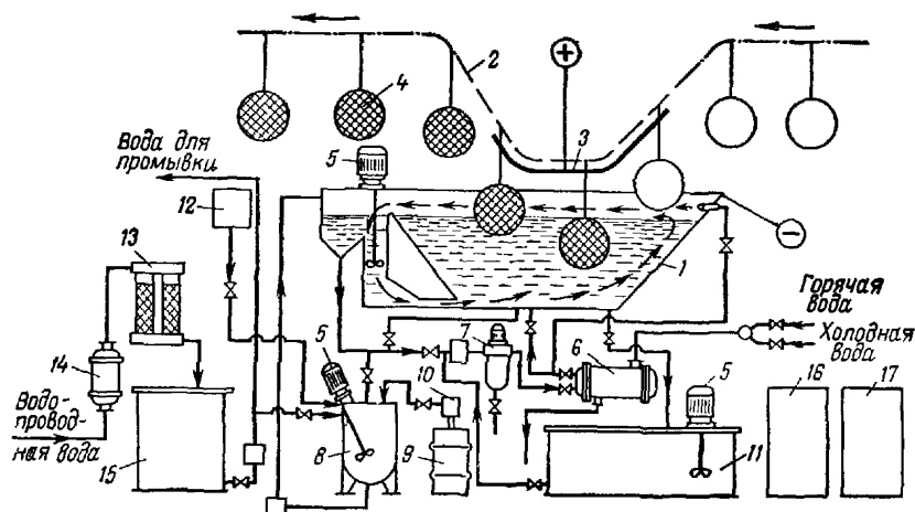
Схема установки электроосаждения:
