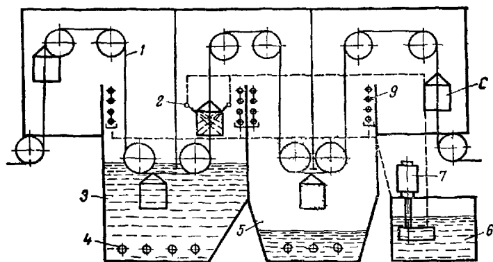
Рис. 4. Схема установки с конвейером замкнутого типа для серийного производства: 1 — конвейер, 2 — форсуноки; 3 — ванна для обезжиривания в жидкости; 4 — нагреватель; 5 — ванна для обезжиривания в парах; 6 — бак с трихлорэтиленом, 7 — насосная станция; 8 — изделие; 9 — холодильник.
