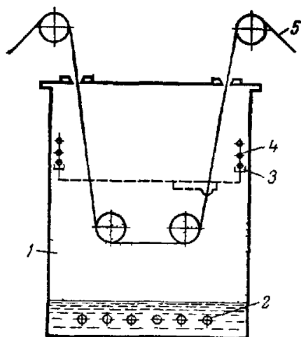
Рис. 1. Схема установки непрерывного обезжиривания металлической ленты, фольги, ткани и т. д.:
