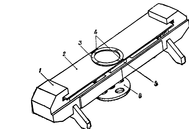
Рис. 4.17. Тарировочное устройство:
