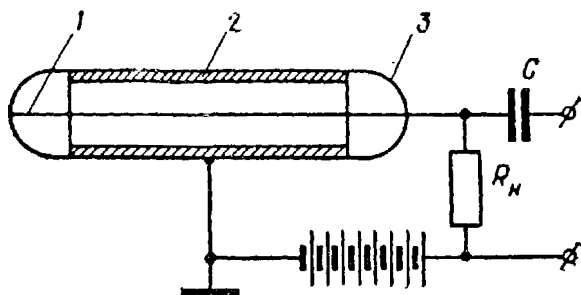
Рис. 2.11. Газоразрядный счетчик:
