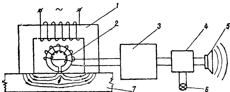
Рис. 4.27. Магнитный щелевой дефектоскоп:
