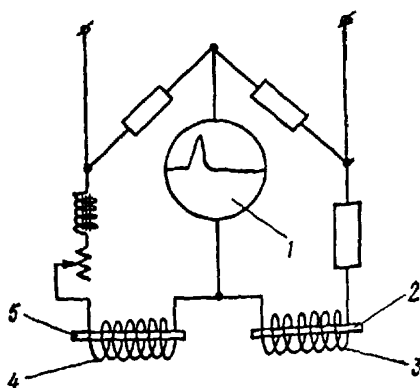
Рис. 4.28. Принципиальная схема электромагнитного индукционного дефектоскопа:
