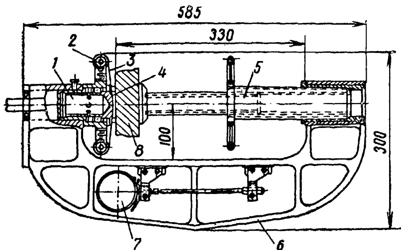
Рис. 3.10. Гидравлический штамп:
