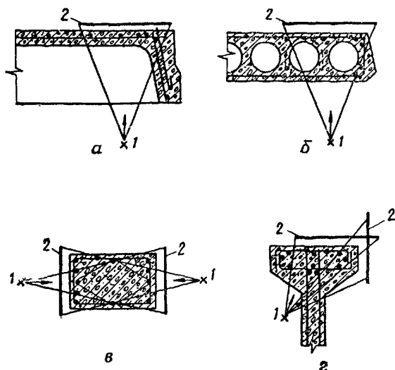
Рис. 3.22. Схемы просвечивания железобетонных конструкций: а — ребристый настил; б — многопустотный настил; в — колонна; г — односкатная балка; 1 — источник излучения; 2 — кассета с пленкой
