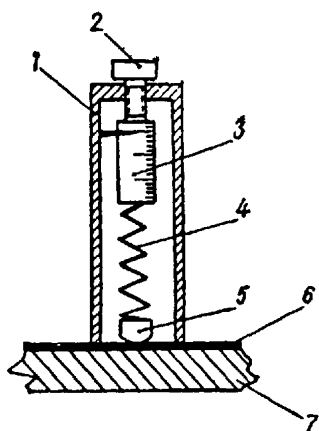
Рис. 4.30. Принципиальная схема простейшего измерителя толщины покрытий:
