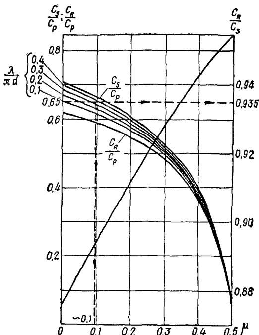
Рис. 5.3. Номограмма Кнопва для определения скорости поперечных волн C_s и коэффициента Пуассона \mu по данным ультразвукового каротажа
