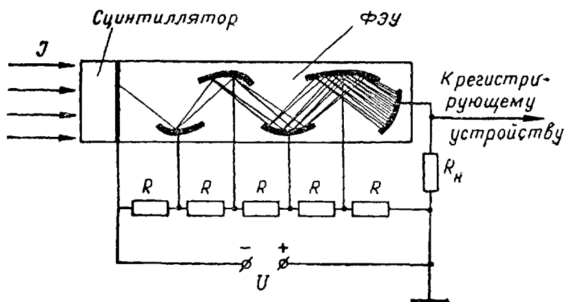
Рис. 2.13. Сцинтилляционный счетчик
