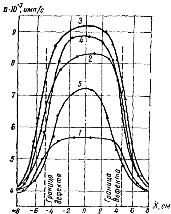
Рис. 3.38. Зависимость скорости счета от координаты датчика при ширине дефекта 9,2 см:
