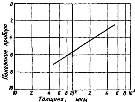
Рис. 4.32. Тарировочный график
