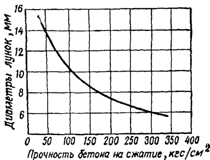
Рис. 3.11. Тарировочный график, построенный по испытаниям молотком И. А. Физделя
