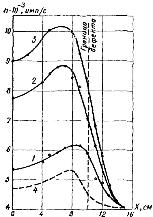
Рис. 3.39. Зависимость скорости счета от координаты датчика при ширине дефекта более 15 см:
