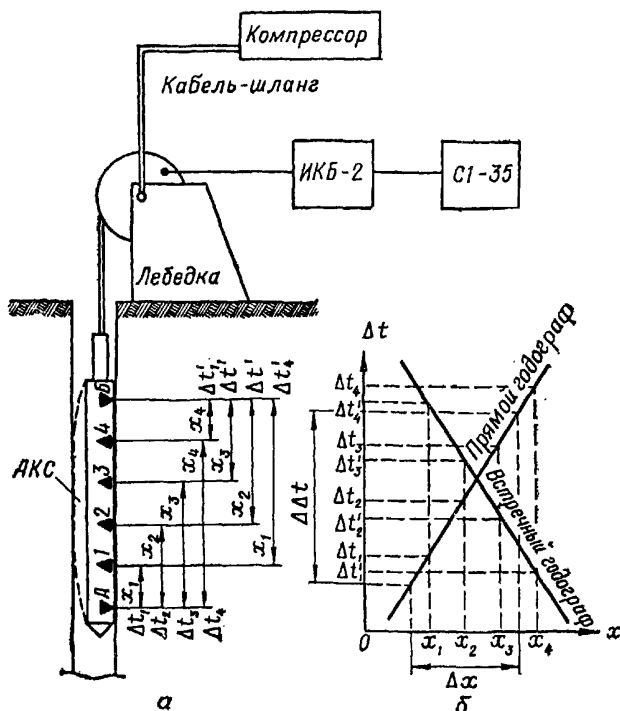
Рис. 5.1. Ультразвуковой каротаж скважин: а — схема каротажа; б — гидрографы скоростей; А, Б — излучатели; 1, 2, 3, 4 — приемники излучения
