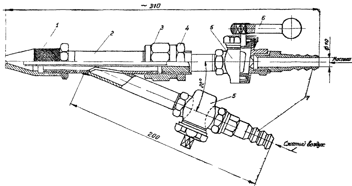
Рис.3. Схема форсунки для нанесения эпоксидно-дегтевого состава: 1- сопло; 2- двойник; 3- муфта; 4- контргайка; 5- ручка ; 6 - ручка; 7- ниппели (размеры в миллиметрах).
