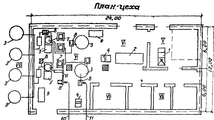
Схема цеха приготовления битумно-каучуковых мастик:
