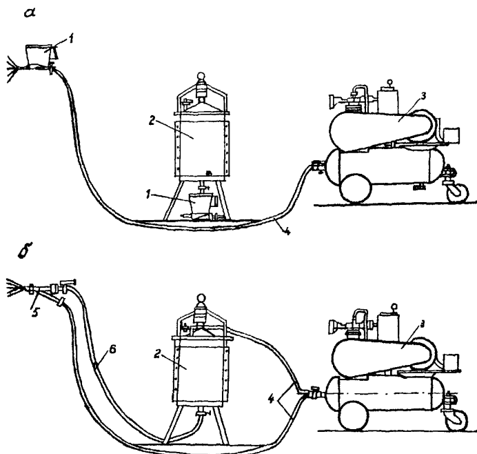
Рис.2. Схема установки для нанесения базу- лонной гидроизоляции при подаче рабочего состава двумя способами: а- бесшланговый; б- шланговый;
