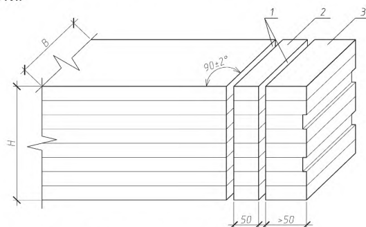
Рисунок 5 — Схема выпиливания заготовки для образцов на послойное скалывание
