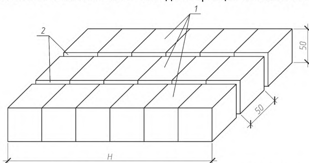
Рисунок 5 — Схема выпиливания заготовки для образцов на послойное скалывание
