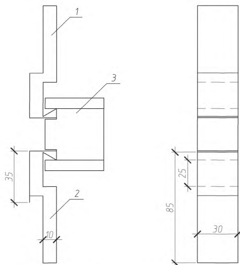
1 – верхняя скоба; 2 – нижняя скоба; 3 – образец
