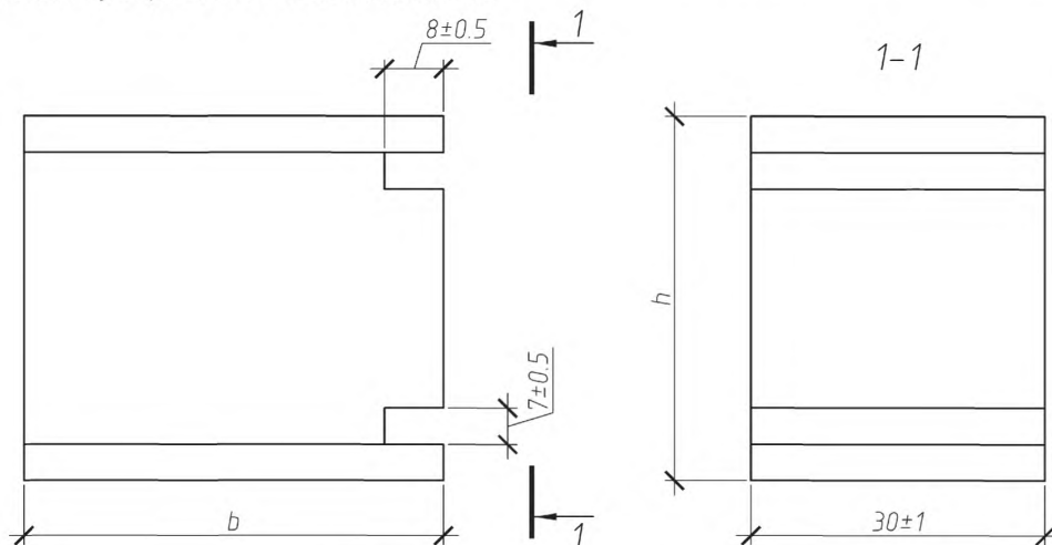
Рисунок 12 – Форма и размеры образца для испытания
