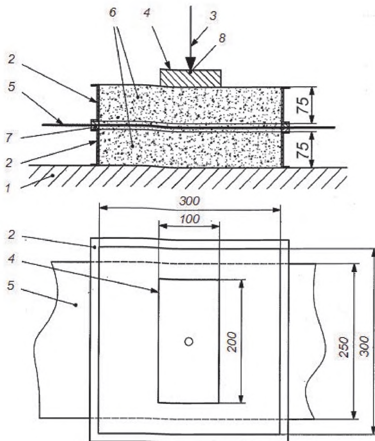
Рисунок А.1 – Схема испытательной установки
