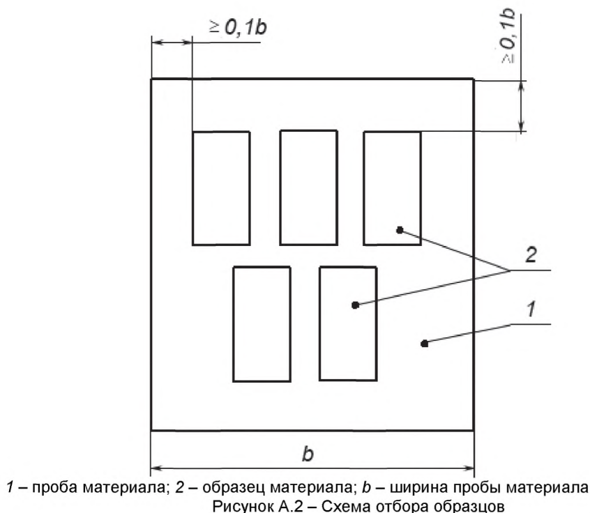
Рисунок А.2 – Схема отбора образцов
