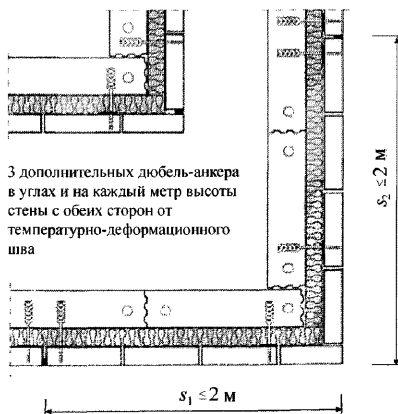
Рисунок 59 – Дополнительные дюбель-анкеры
