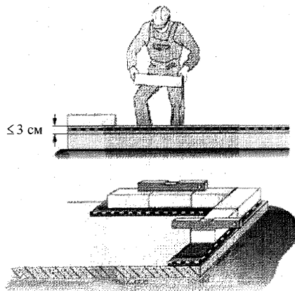
Рисунок 27 – Выполнение опорного ряда кладки
