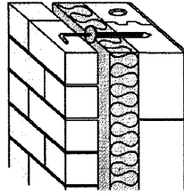
Рисунок 56 – Стержневые связи с прижимными влагоотводящими шайбами
