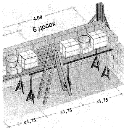
Рисунок 14 – Переставные леса, размеры в м
