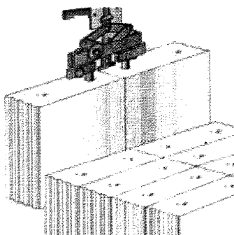
Рисунок 46 – Захват рейфферным захватным устройством двух блоков
