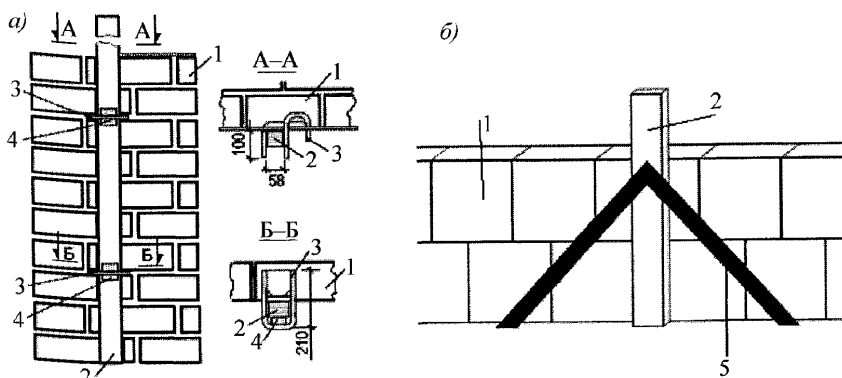
а) – кирпичная кладка на кладочном растворе; б) – крупноблочная кладка на растворе для тонкошовной кладки; 1 – кладка; 2 – маячная рейка (порядовка); 3 – держатель рейки; 4 – клин; 5 – установочная рейка
