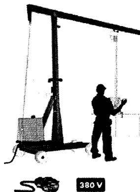
Рисунок 17 – Кран малой грузоподъемности
