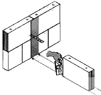
Рисунок 41 – Нанесение раствора для тонкошовной кладки на примыкающий элемент
