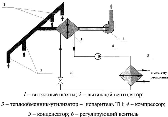
Рисунок 2 – Схема теплообменника-утилизатора теплоты вентиляционных выбросов с встроенным испарителем ТН
