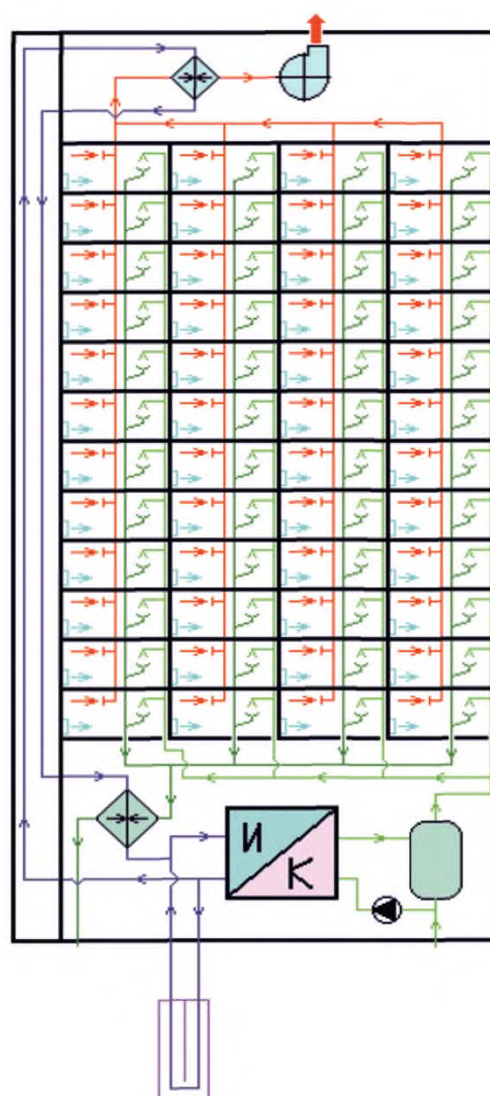
Рисунок 9 – Комбинированное использование теплоты вентиляционных выбросов, грунта и канализационных стоков жилого дома
