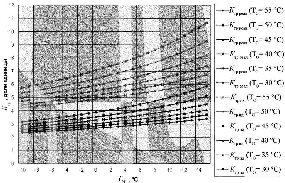
Рисунок А.2 – Типичный вид зависимости идеального и реального коэффициента трансформации энергии парокompрессионных тепловых насосов от температур испарения и конденсации хладагента
