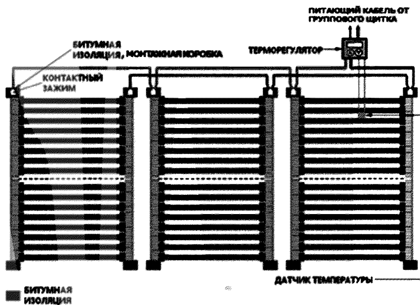
Рисунок Е.2 – Схема подключения листов нагревательной пленки к терморегулятору
