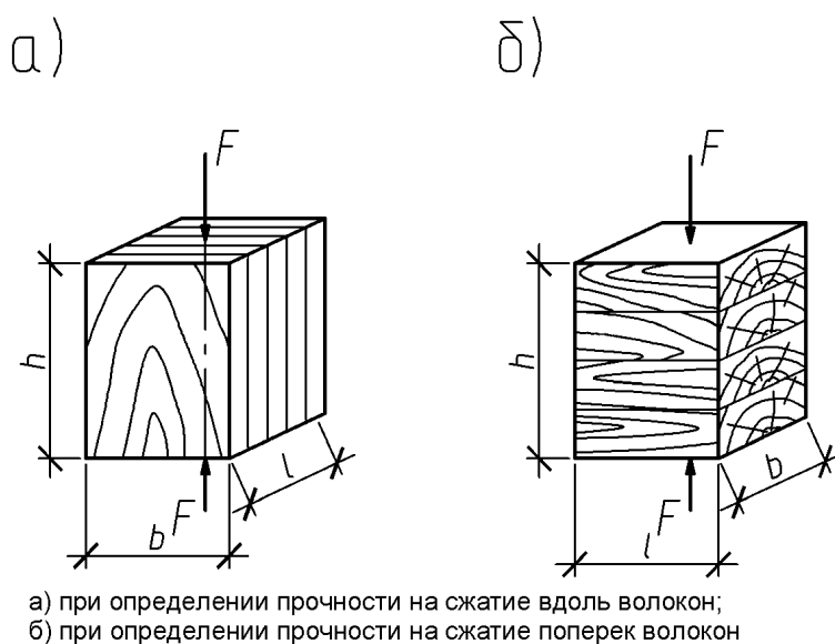
Рисунок Б.3 – Обозначение размеров и схемы испытаний образцов клееных элементов
