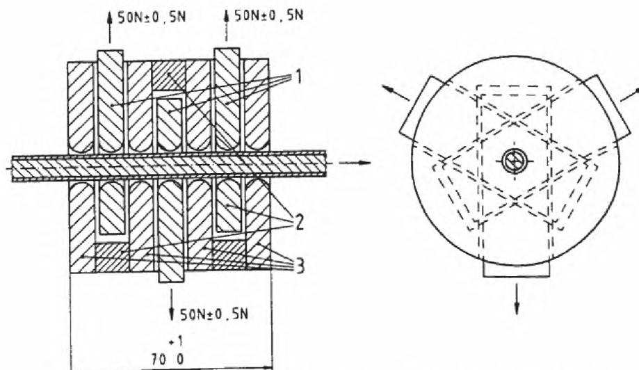
1 – движущиеся пластины; 2 – пространство; 3 – закрепленные пластины
