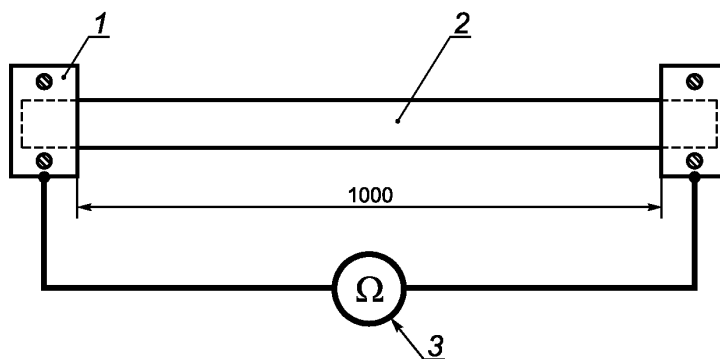
1 — разборные сдвоенные медные пластины; 2 — испытуемый образец; 3 — омметр
