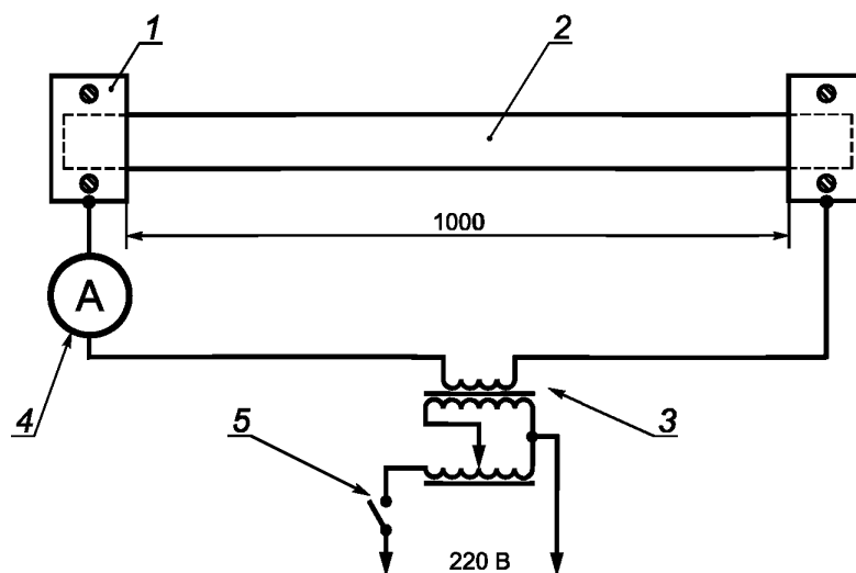
1 — разъёмные сдвоенные медные пластины; 2 — испытуемый образец; 3 — регулируемый источник напряжения; 4 — амперметр; 5 — выключатель
