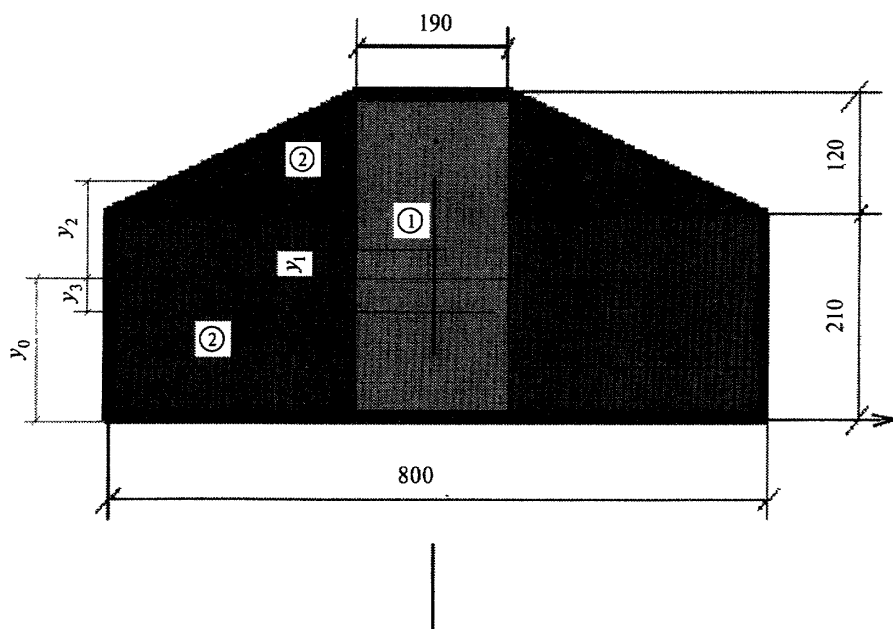
Нейтральная ось и расстояния от нее до центров тяжести элементов сечения балки
