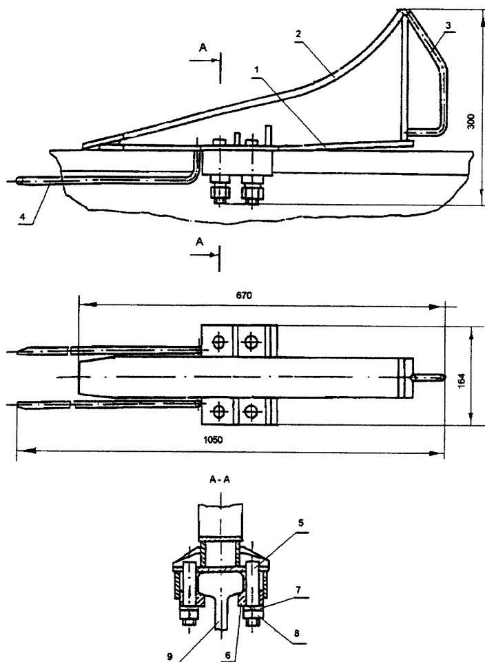
Рисунок 5 – Крепление тупикового упора к рельсу
