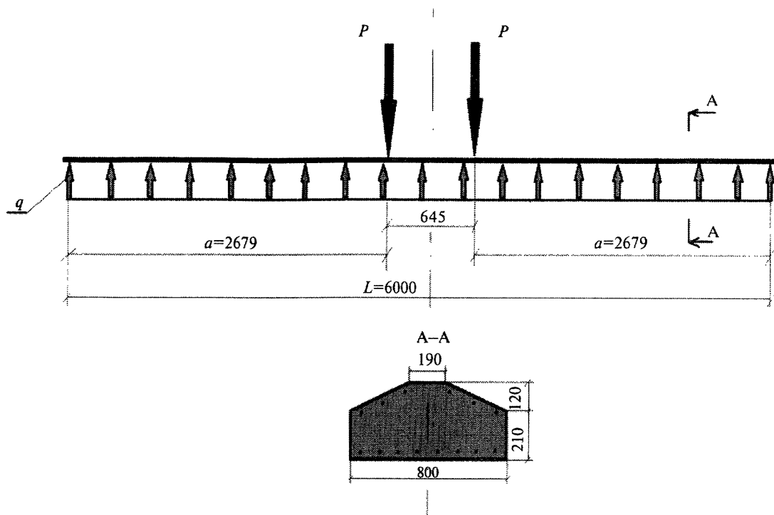
Расчетная схема балки
